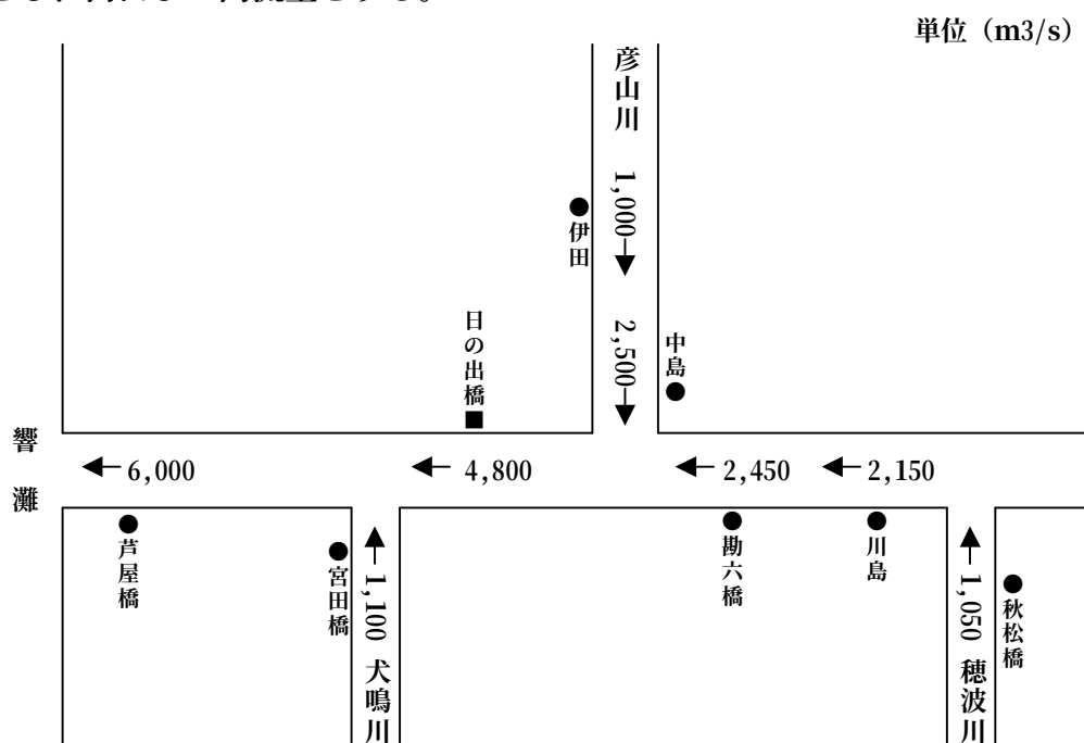
図 6-1 遠賀川計画高水流量図
