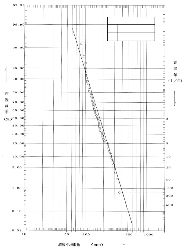
日の出橋地点基準における雨量確率評価
