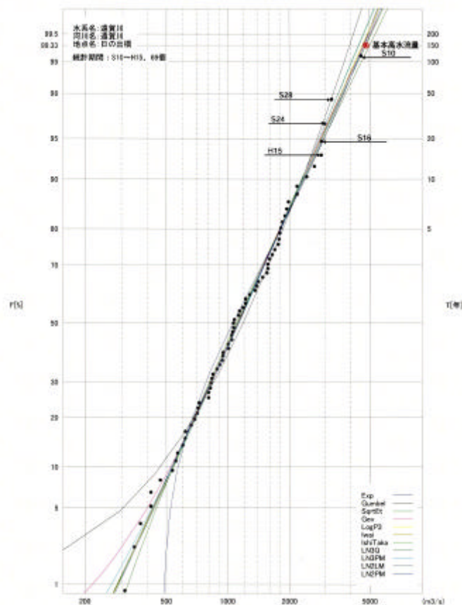
日の出橋地点流量確率計算結果図
