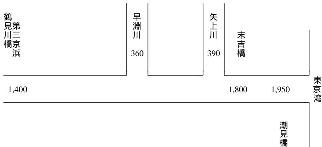
計画高水流量配分図
