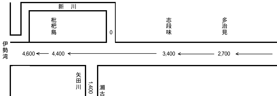
庄内川計画高水流量図 (単位： \text{m}^3/\text{s} )
