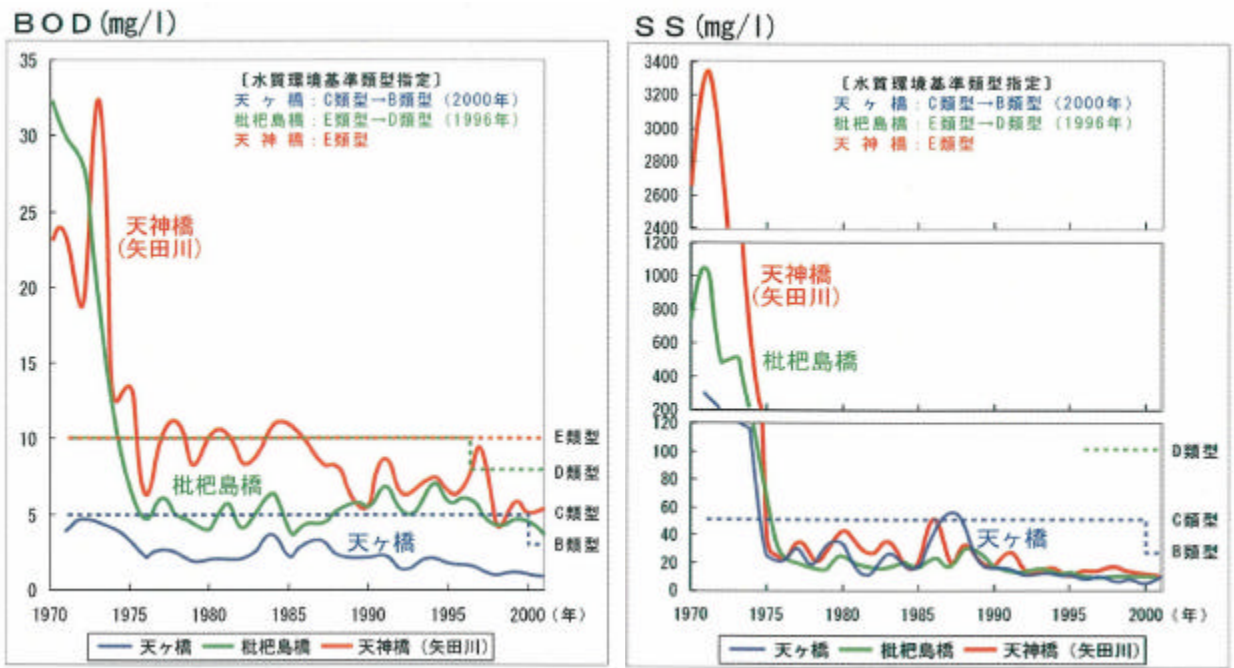
BOD、SSの変化状況
