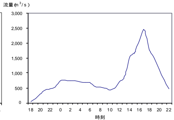
図 4-3 流量ハイドログラフ
