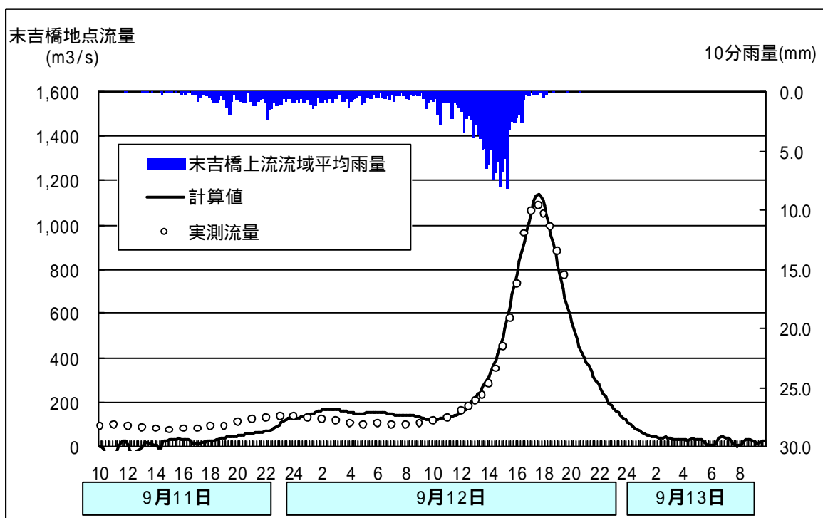
図 4-2 昭和 57 年 9 月洪水再現計算結果（末吉橋地点）
