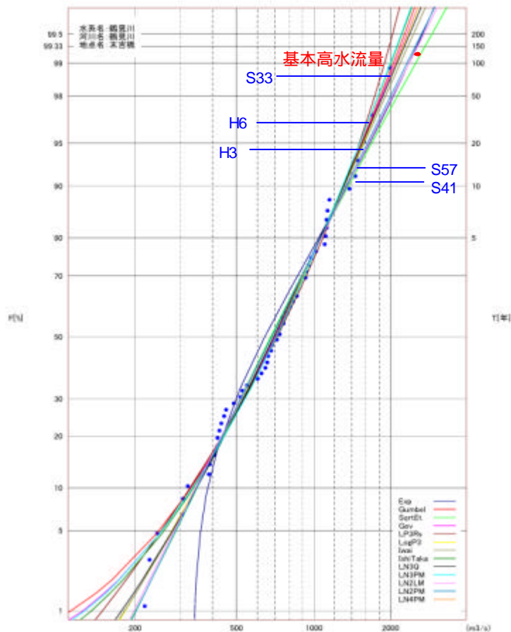
図 4-7 末吉橋地点流量確率計算結果図
