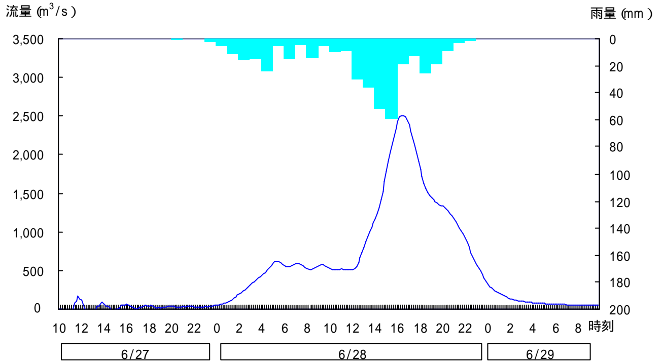
図 4-8 昭和 41 年 6 月型ハイドログラフ (末吉橋地点)
