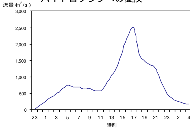
図 4-3 流量ハイドログラフ
