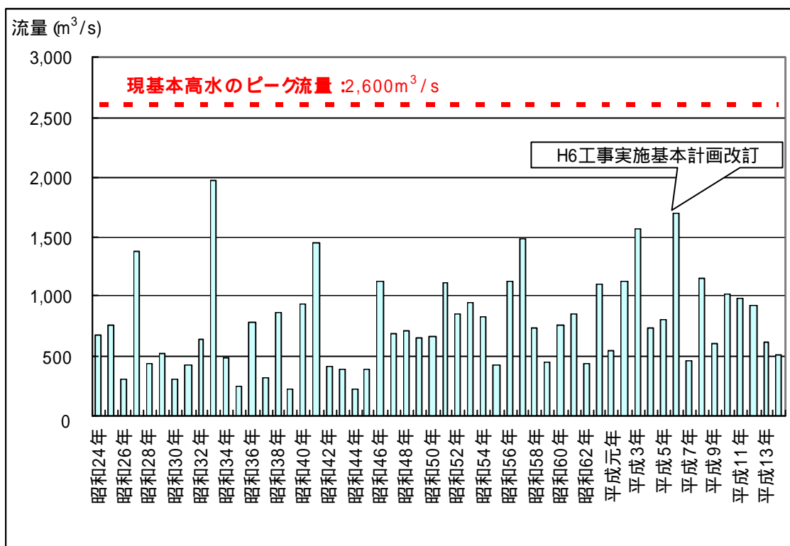
図 4-6 末吉橋地点年最大流量
