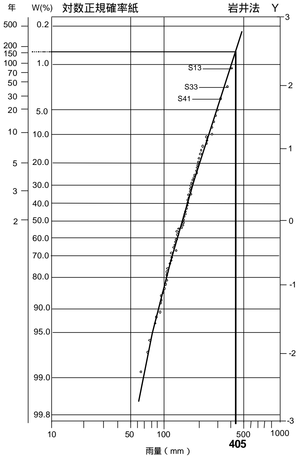
図 4-1 末吉橋地点における雨量確率評価 (2 日雨量)
