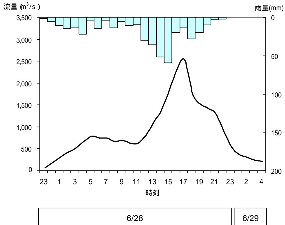
図 4-4 昭和41年6月型ハイドログラフ（末吉橋地点）
