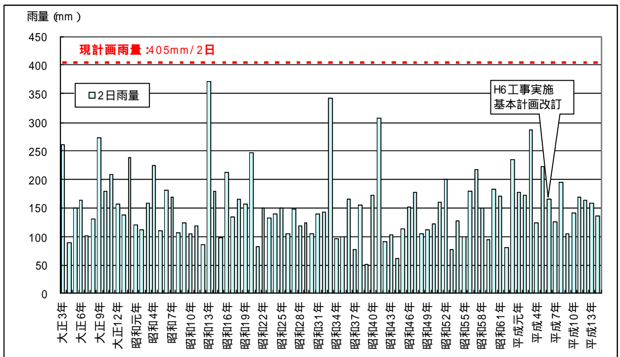
図 4-5 流域平均年最大2日雨量
