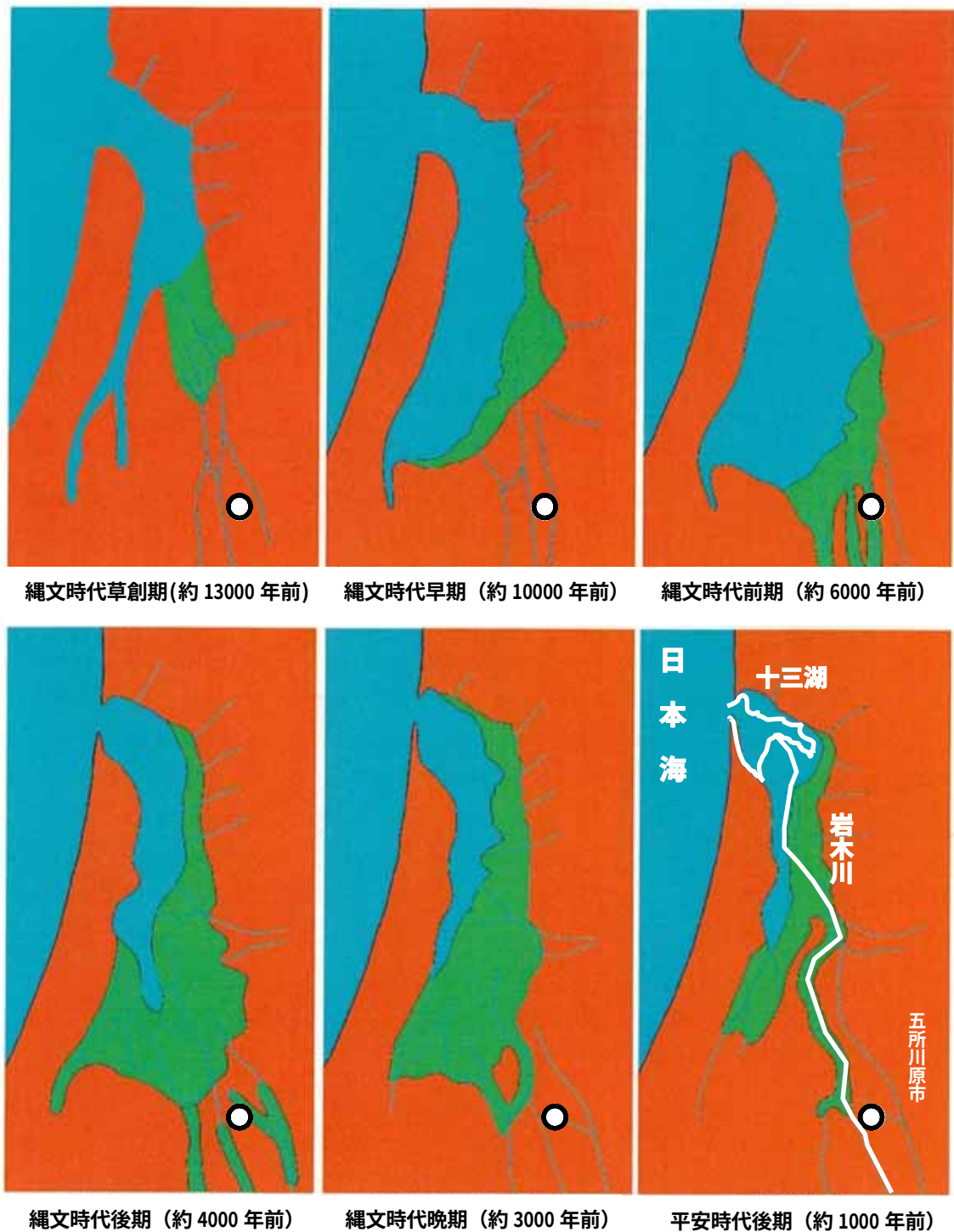
図 1-7 縄文海進図
