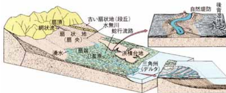
図 1-5 地形概略図
