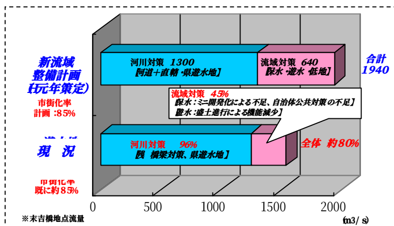
図 4-3-11 新流域整備計画と現況との比較による河川・流域対策の達成状況
