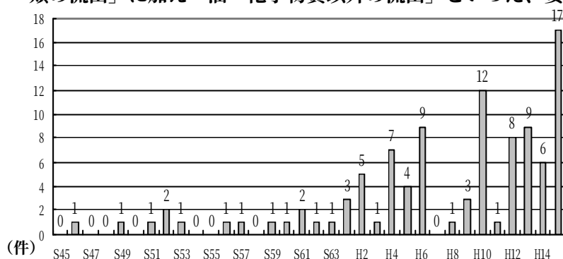
図 9-4-4 水質事故の水位 出典：京浜河川事務所
