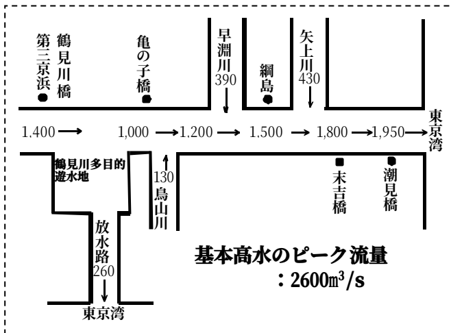
図4-3-9 平成6年 流量配分図(単位: \text{m}^3/\text{s} ) 出典: 京浜河川事務所
