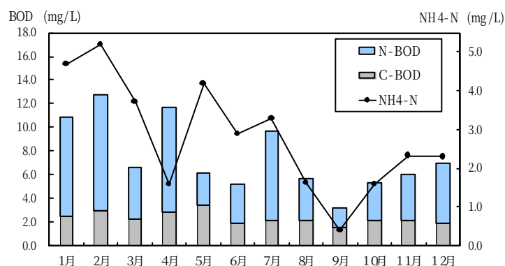
図 6-3-9 亀の子橋におけるBODの内訳 (平成 15 年) 出典：京浜河川事務所
