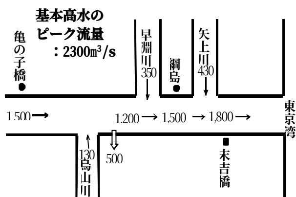
図 4-3-4 昭和 49 年 流量配分図 (単位: \text{m}^3/\text{s} ) 出典: 京浜河川事務所
