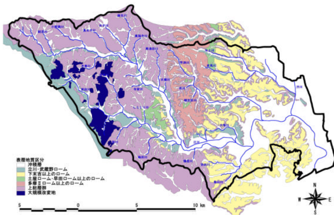
图 1-3-1 地质图
