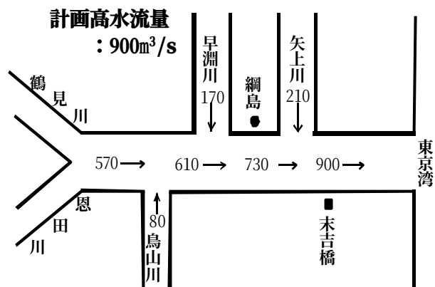
図 4-3-3 昭和 43 年 流量配分図 (単位: \text{m}^3/\text{s} ) 出典: 京浜河川事務所
