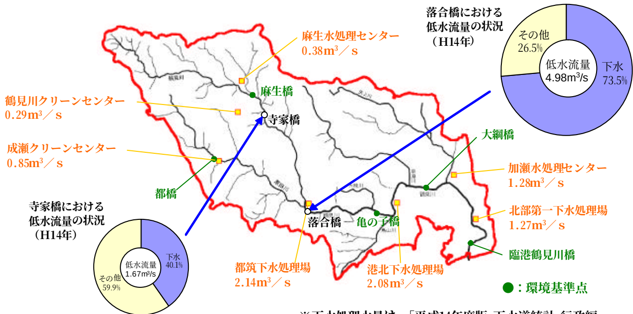
図 6-2-1. 下水処理水の流入状況 (H14 年度)
