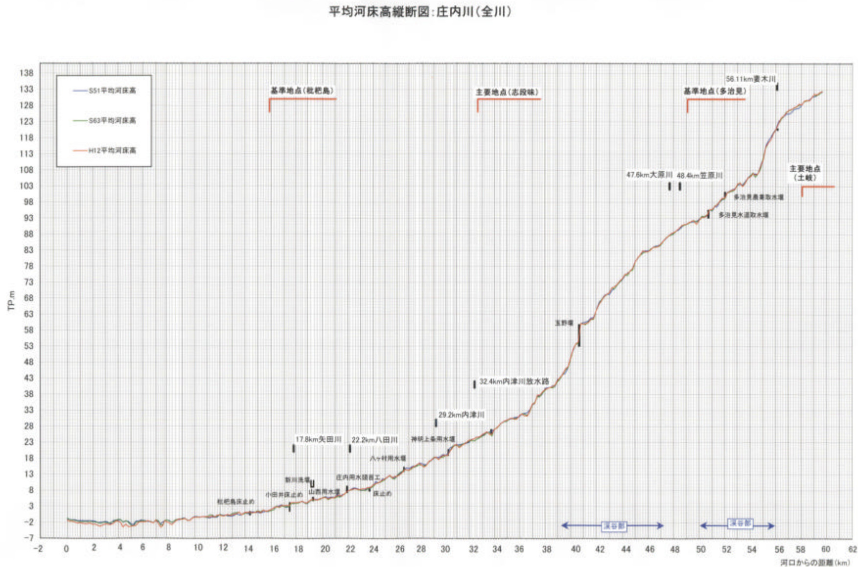
図-8.8 平均河床高縦断面図の経年変化
