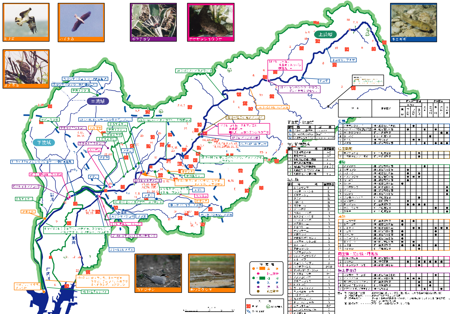
図-2.4 庄内川流域の自然環境(動物)
