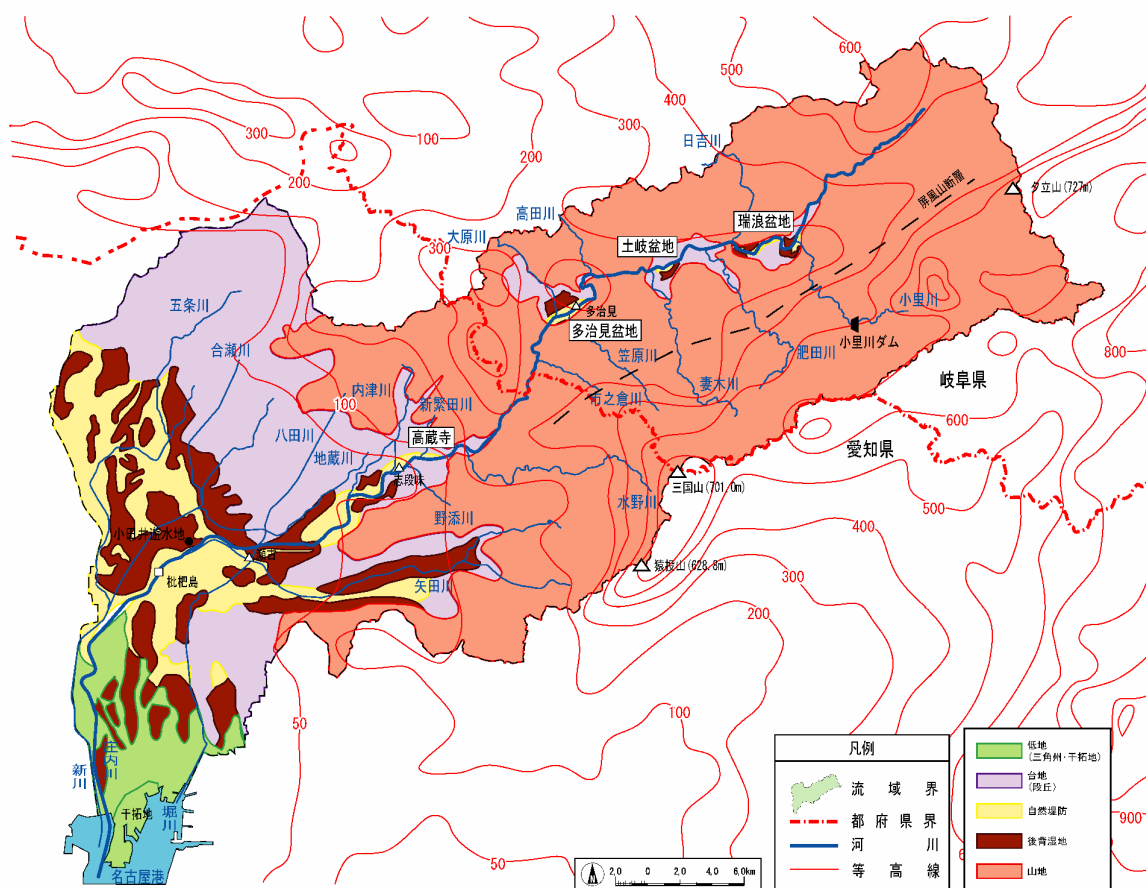
図-1.5 庄内川流域地形区分図
