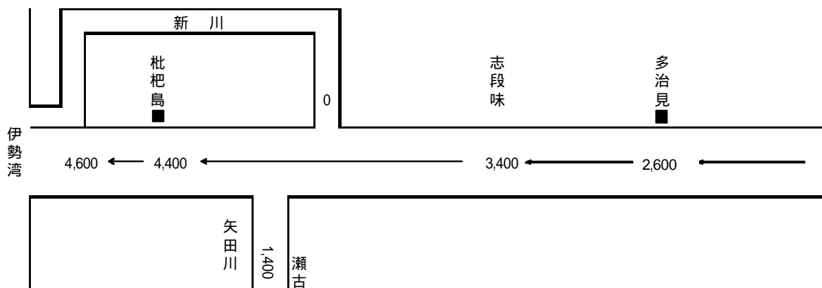
庄内川計画高水流量図 (単位：m 3 /s)
