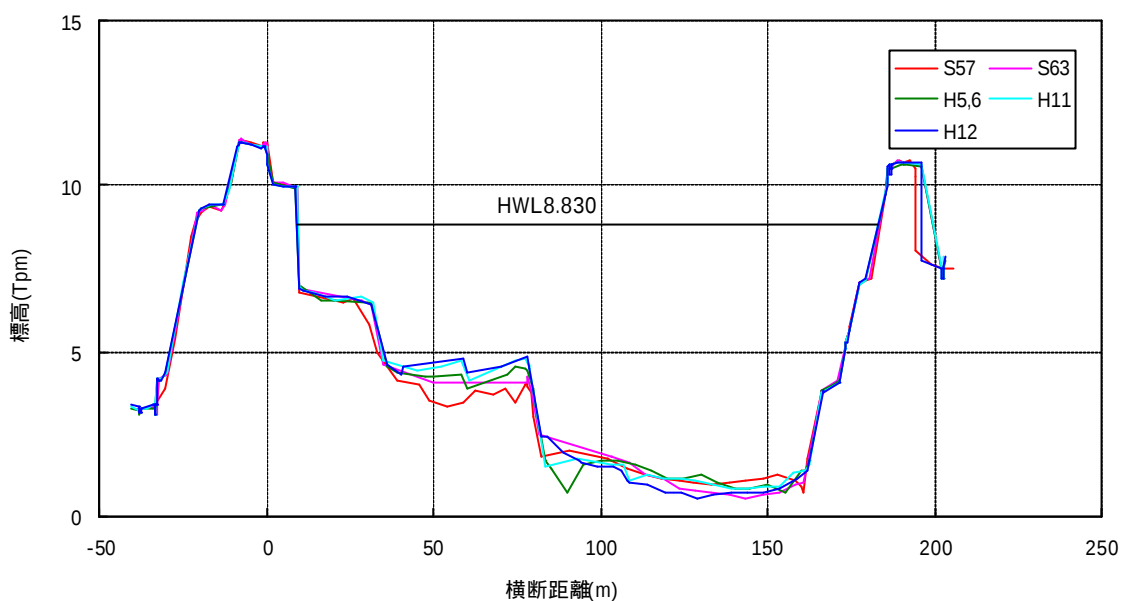
図-8.6 横断形状の経年変化 (15.8k)
