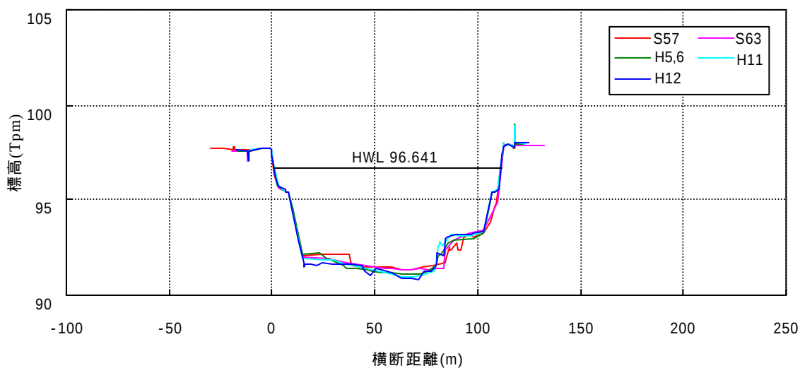
図-8.6 横断形状の経年変化 (15.8k)
