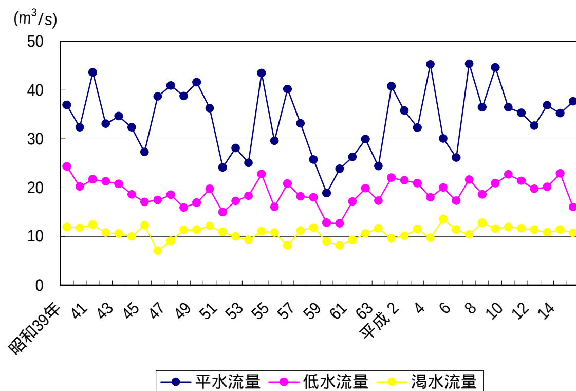
図 6-2 富川地点流況経年変化図
