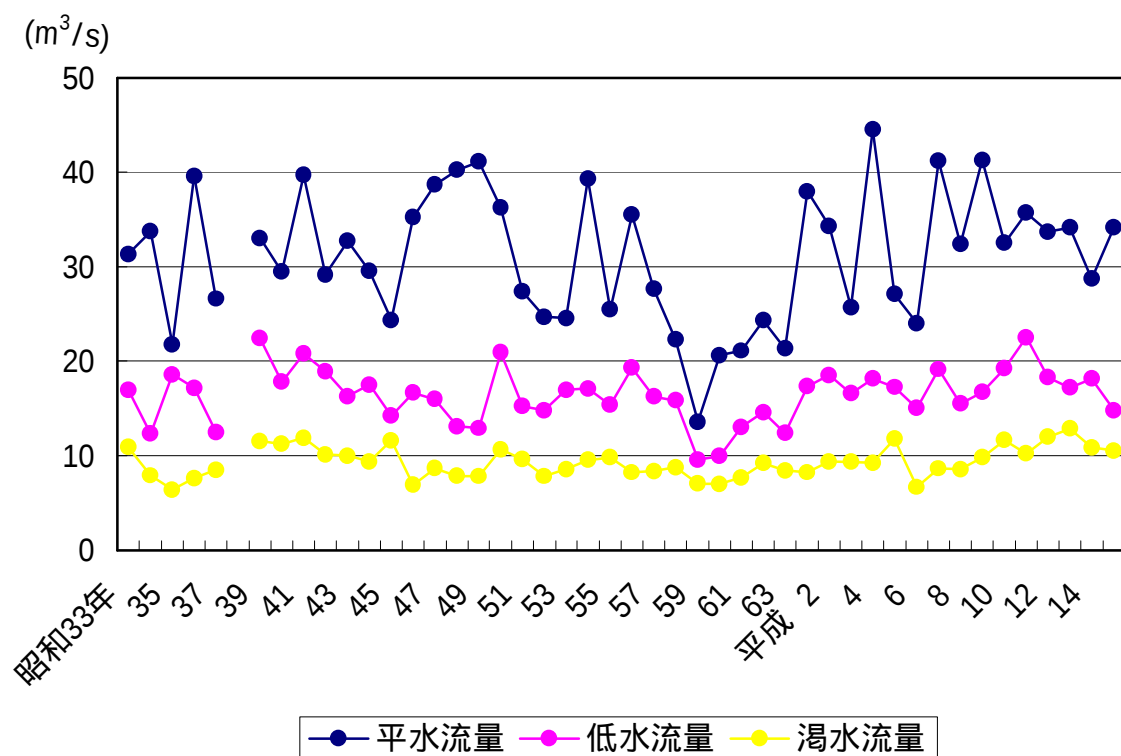
図 6-1 平取地点流況経年変化図
