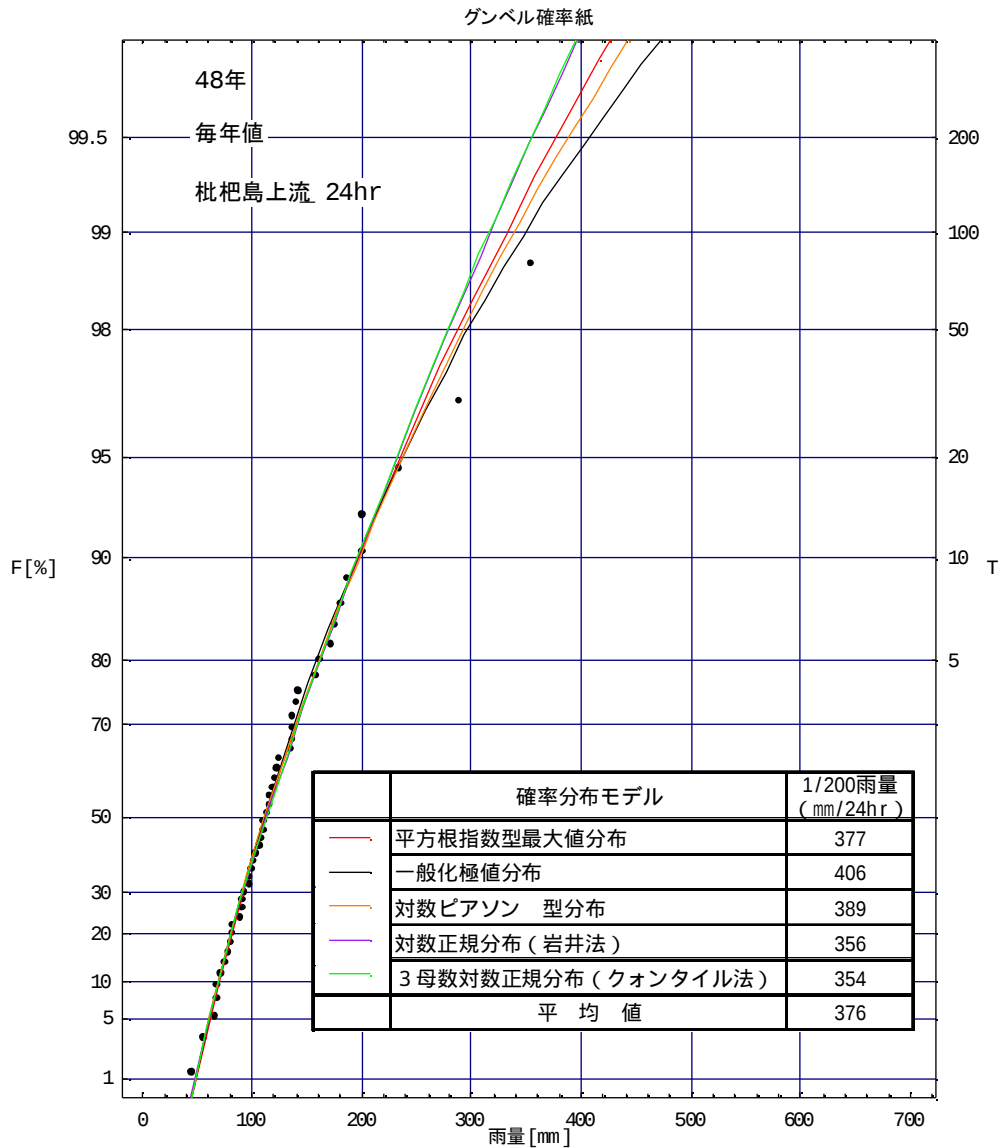
図 4 - 5 基準地点枇杷島における雨量確率図 (S30～H14：48 ケ年)
