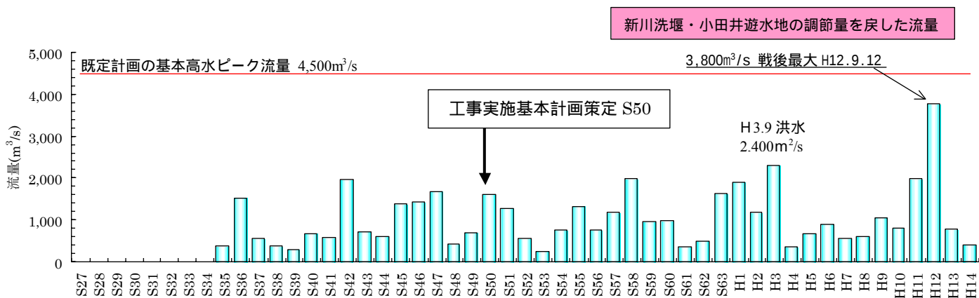
図 4 - 3 枇杷島地点 年最大流量
