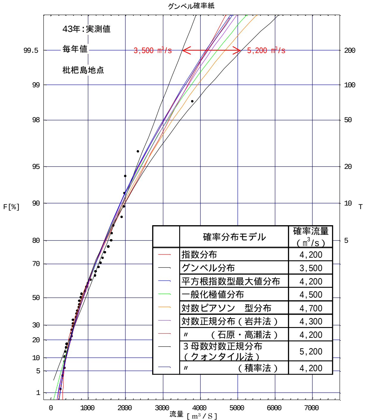
図 4 - 9 基準地点枇杷島における流量確率図（S35～H14：43 ケ年）
