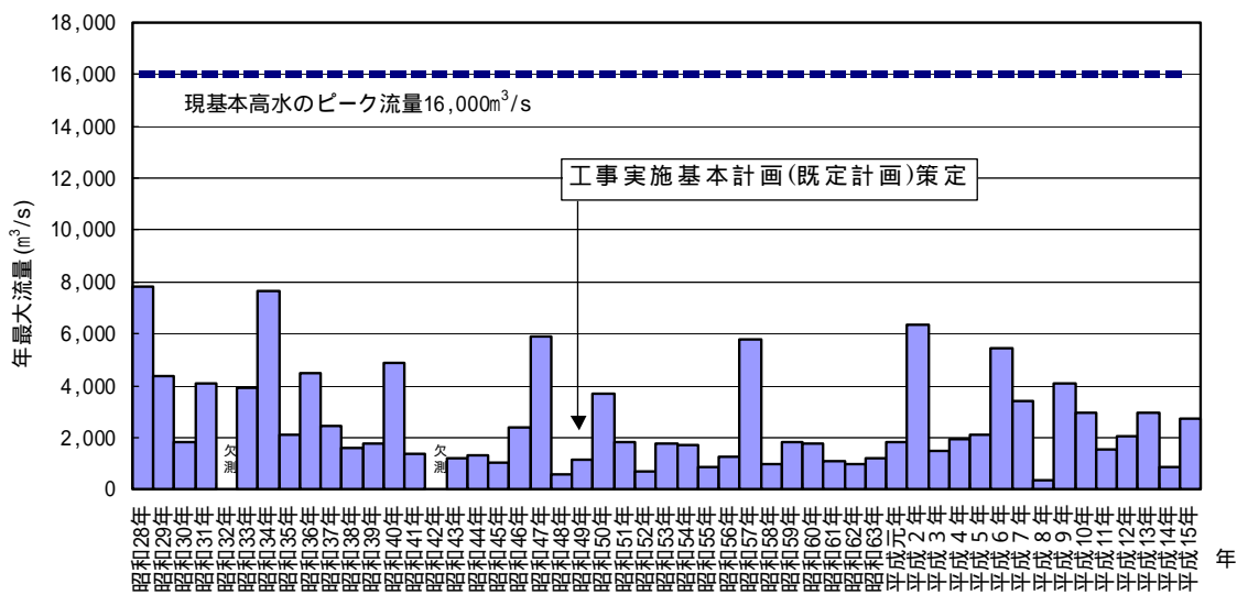
図4-5 年最大流量（船戸地点）
