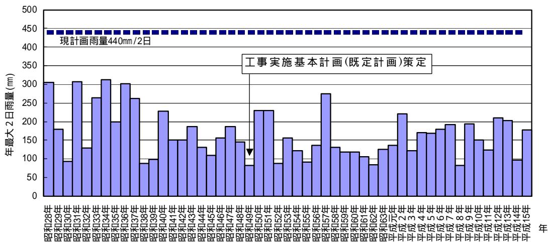
図4-6 年最大2日雨量（船戸地点上流域平均）
