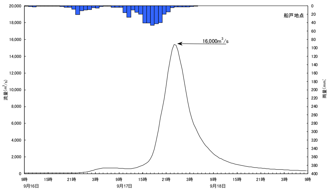
図 4 - 1 0 昭和 40 年 9 月型ハイドログラフ ( 船戸地点 )
