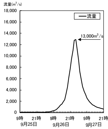
図 4 - 3 ハイドログラフの算定結果
