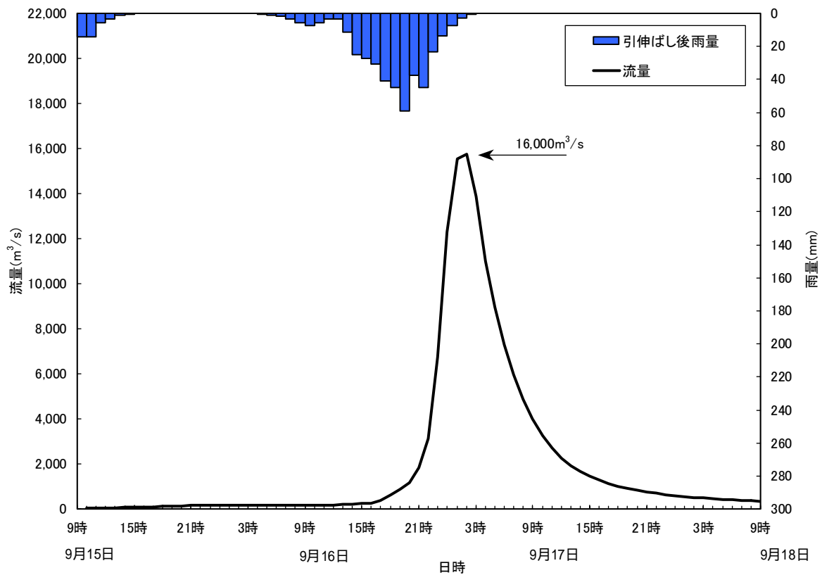
図 4 - 4 昭和47年9月型ハイドログラフ（船戸地点）
