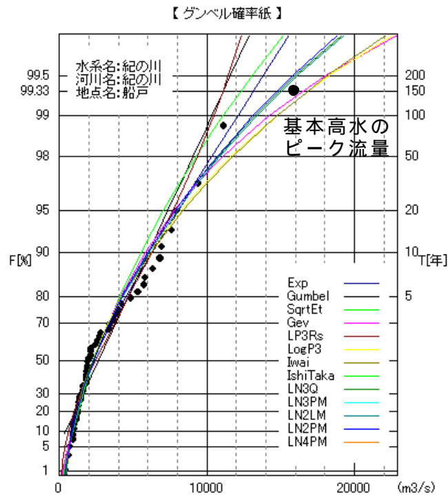
図 4 - 7 船戸地点流量確率計算結果
