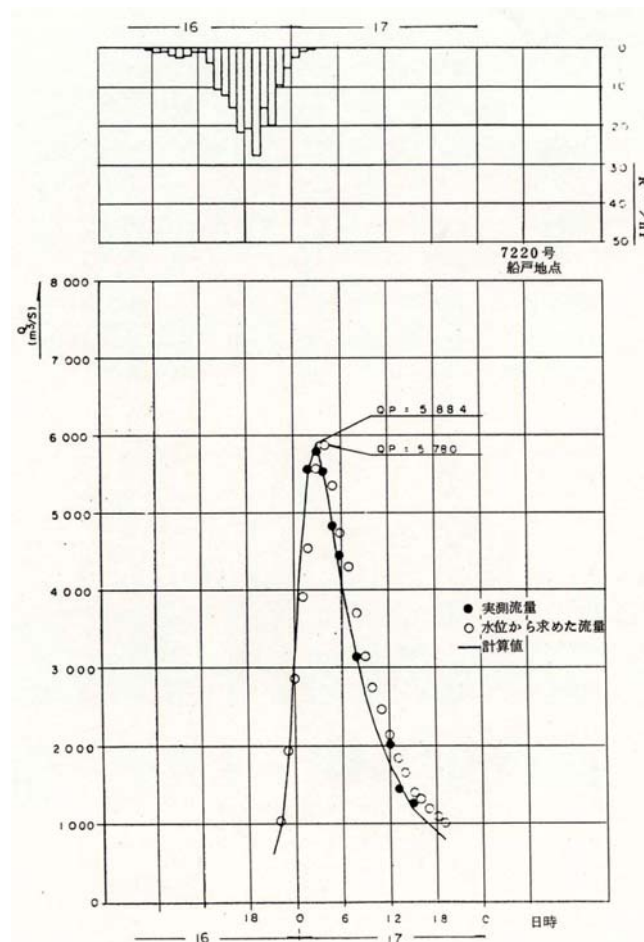
図 4 - 2 昭和47年9月洪水再現計算結果（船戸地点）
