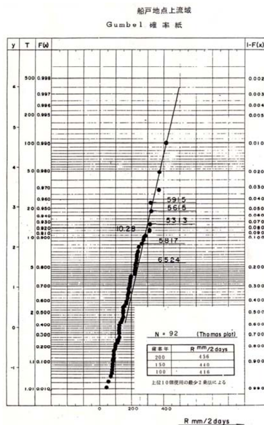
図 4 - 1 船戸地点における雨量確率評価
