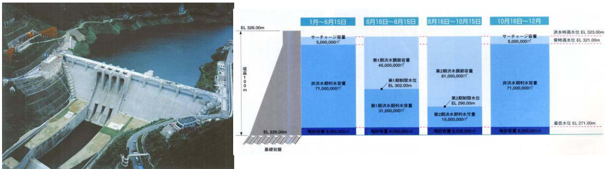
大滝ダム貯水容量配分図
