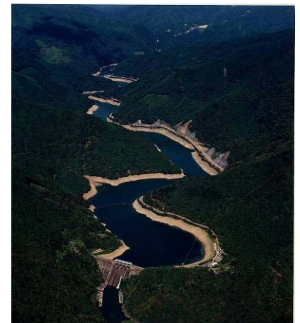
猿谷ダム渇水状況 (平成7年9月：貯水率15.7%)
