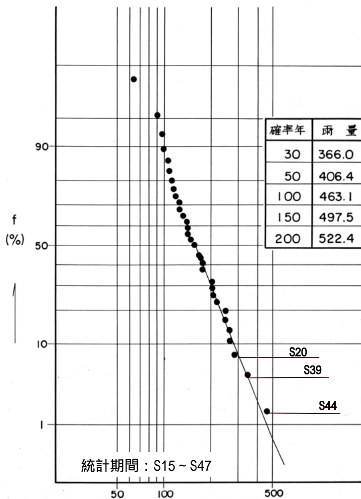
図 4 - 1 瓶岩地点基準における雨量確率評価
