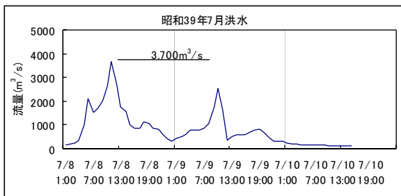
図4 - 4 主要洪水における計画降雨量への引伸ばしと流出計算
