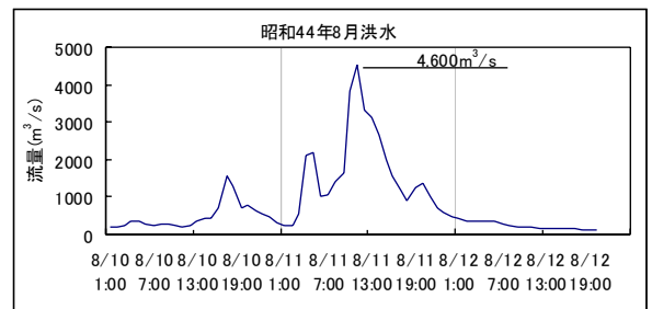
図4 - 4 主要洪水における計画降雨量への引伸ばしと流出計算
