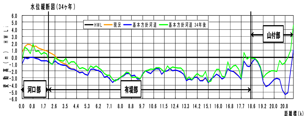
図 - 4 基本方針河道の河床変動予測結果 (直轄管理区間を対象)
