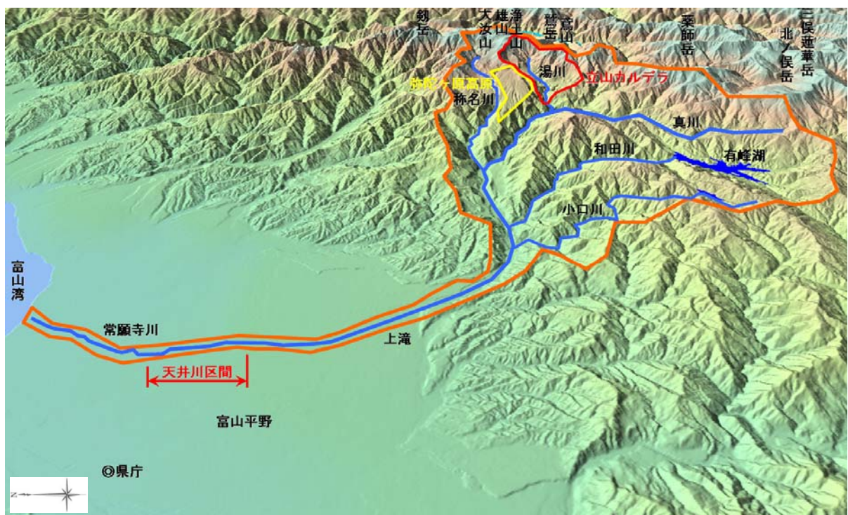
図 1-2 常願寺川流域の地形
