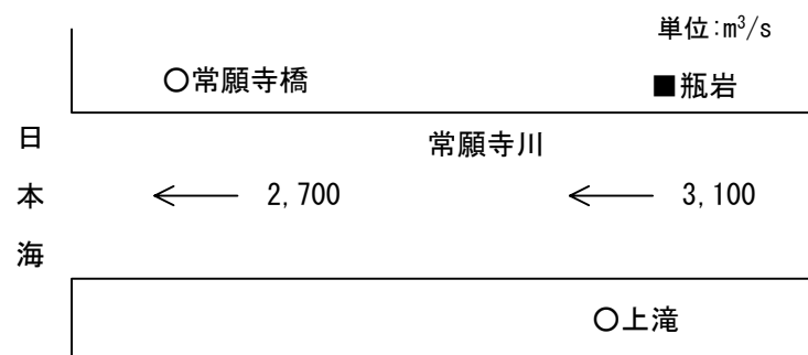
図 4-2-2 計画高水流量図(昭和43年2月7日策定)
