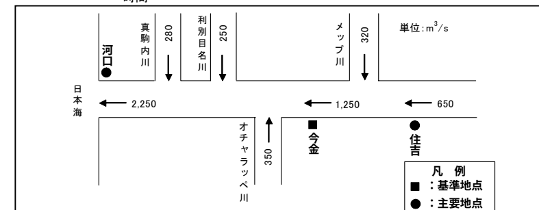
河川整備基本方針における流量配分
