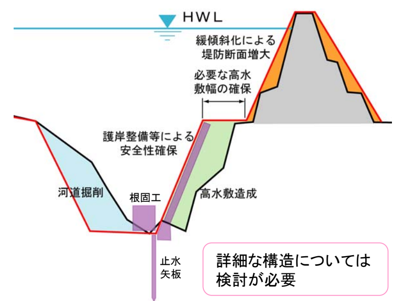
堤体強化対策概念図
