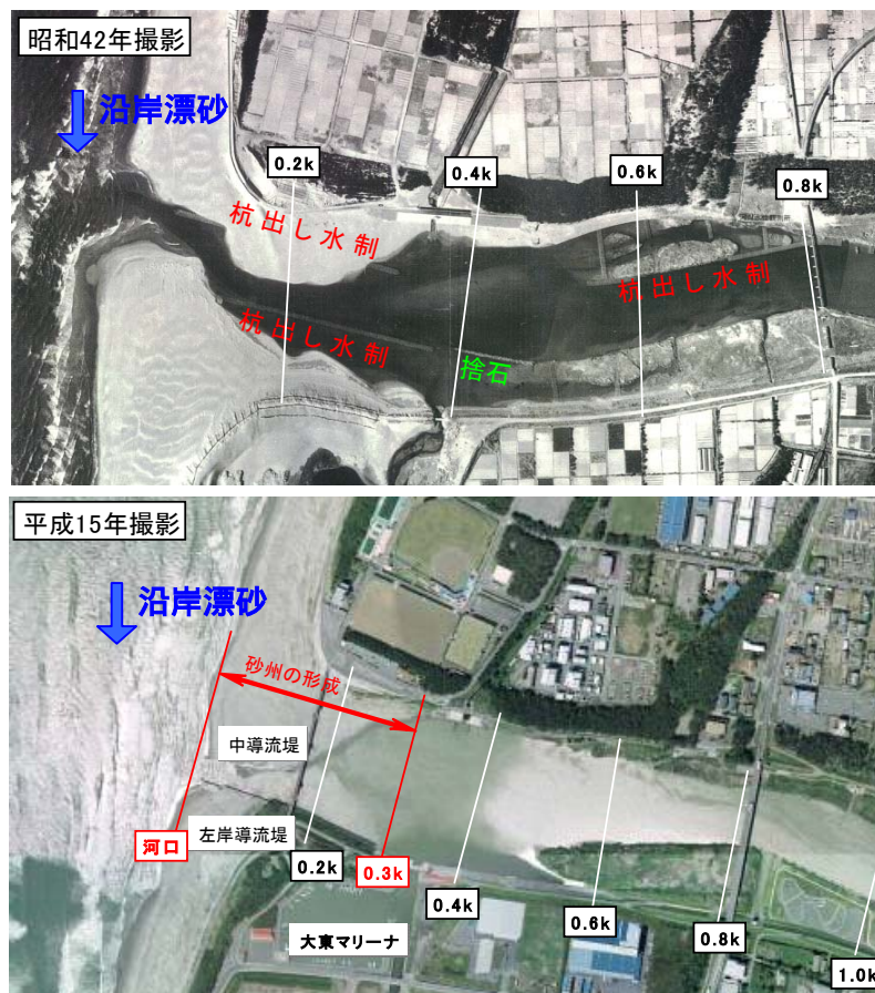
図 3-1 河口部の変遷
