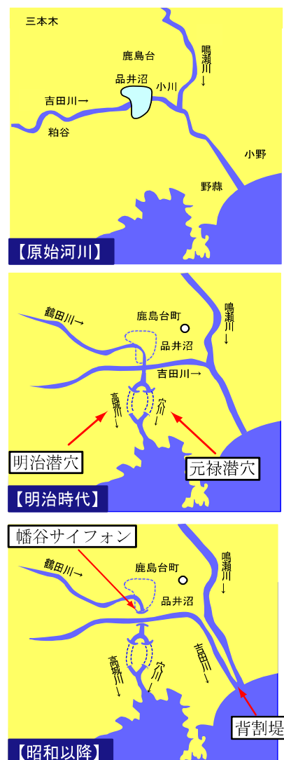
図 3-11 河道の変遷
