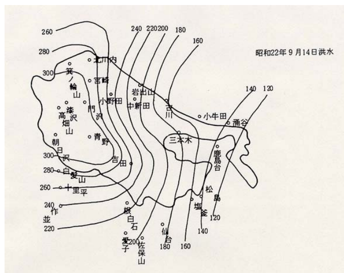
図 3-1 昭和 22 年 9 月洪水等雨量線図
