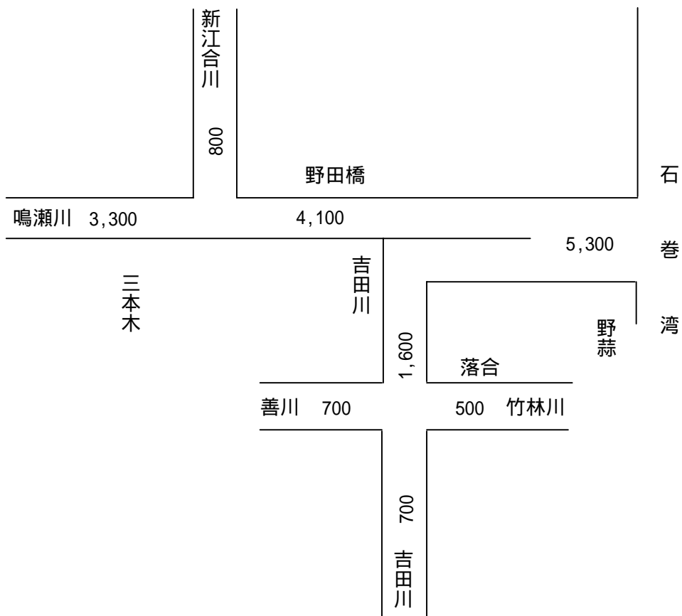
図 6-1 計画流量配分図
