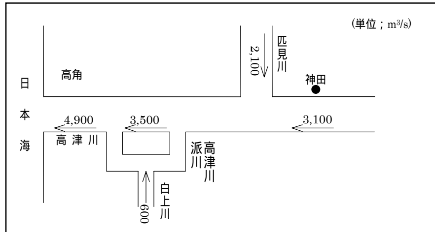
図 6-1 高津川計画高水流量図
