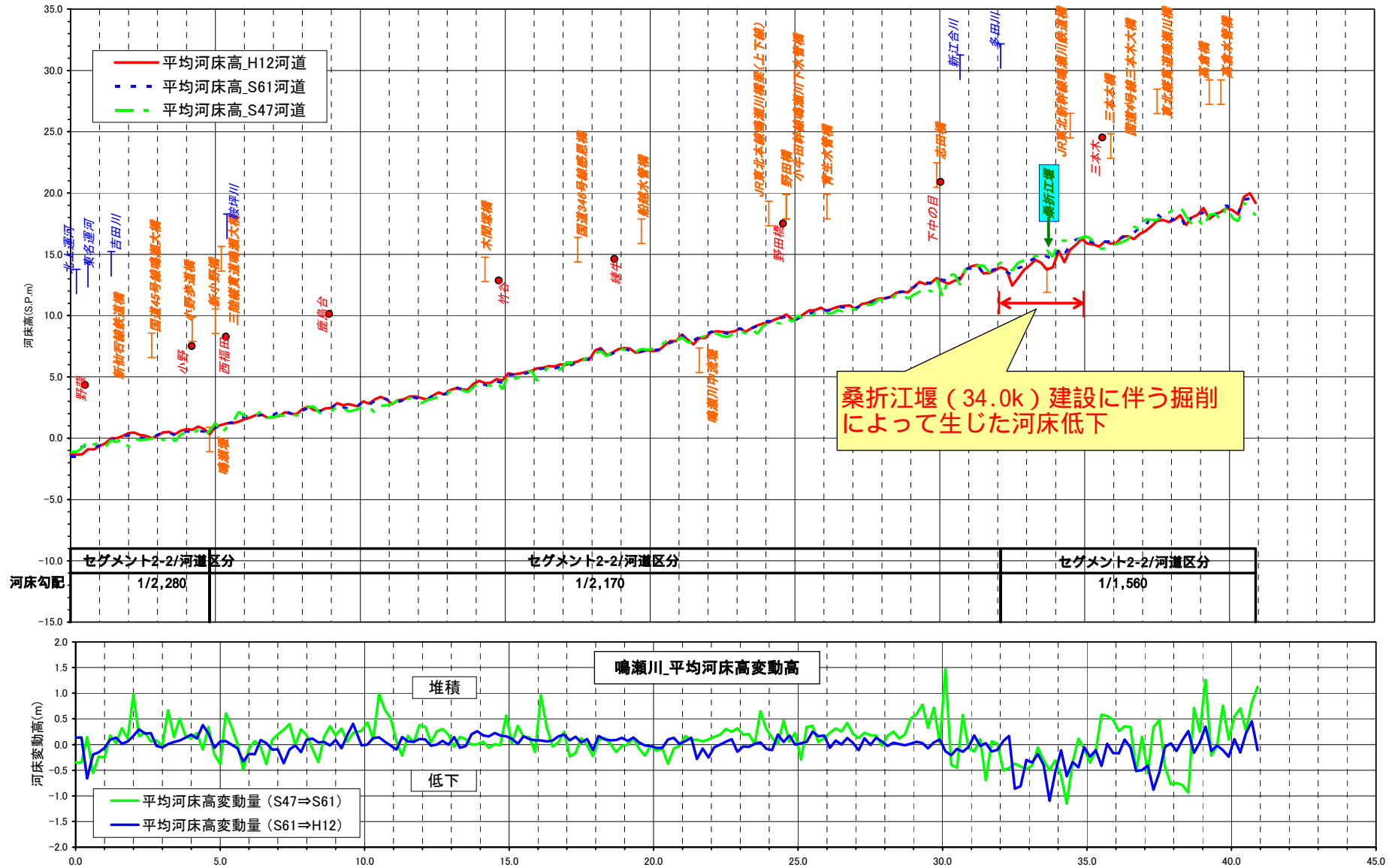
図 2-1(1) 【鳴瀬川】 低水路平均河床高縦断図 (上)、河床変動縦断図 (下)
