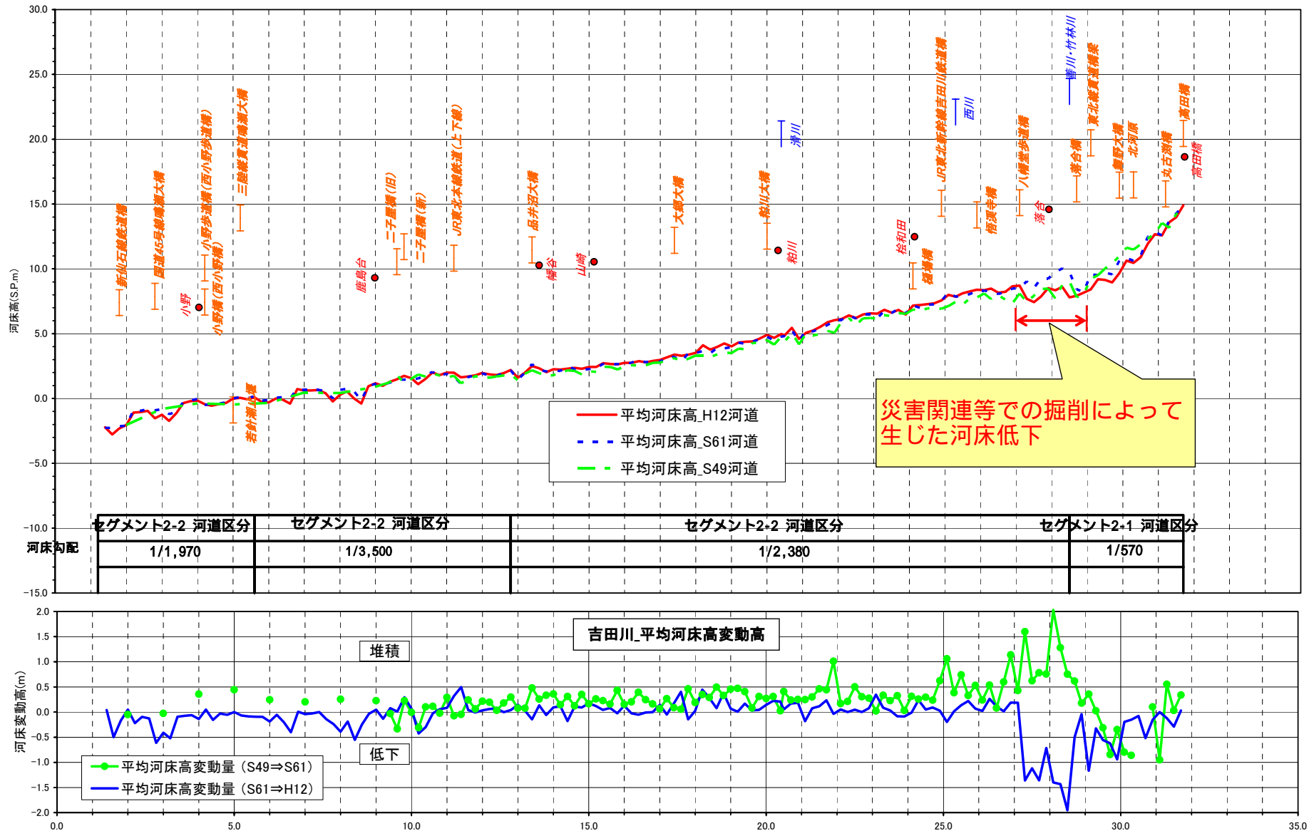
図 2-1(2) 【吉田川】 低水路平均河床高縦断面図(上)、河床変動縦断面図(下)
