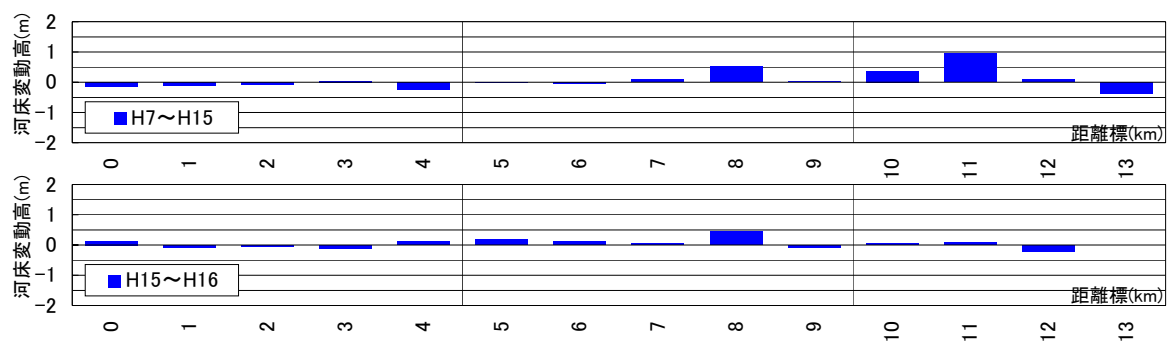
図 2 - 9 河床変動高の経年変化（足羽川）
