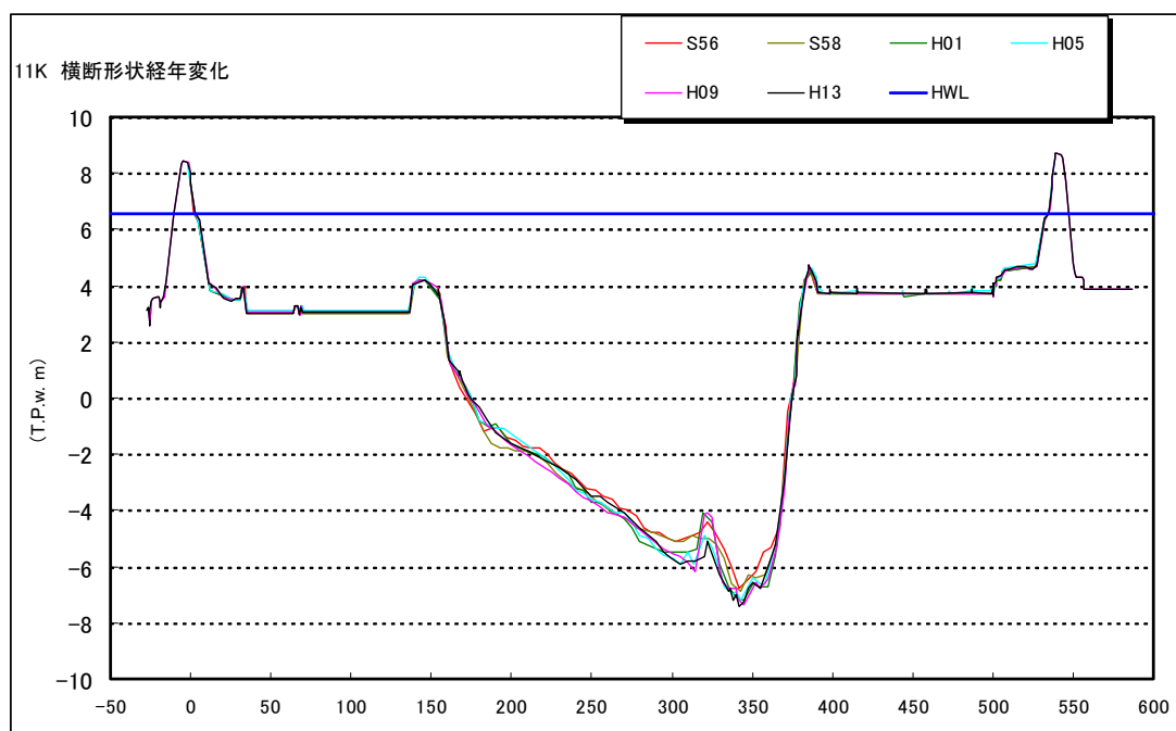
図2-10 九頭竜川（布施田橋上流 11.0k）横断図
