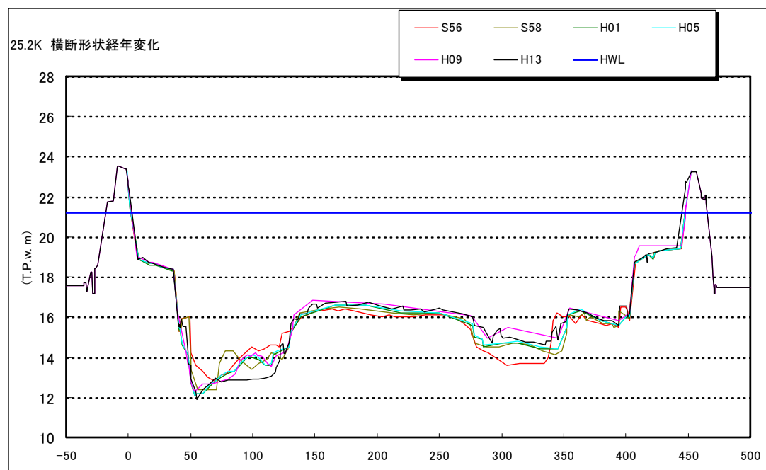
図2-11 九頭竜川（福松大橋下流 25.2k）横断図
