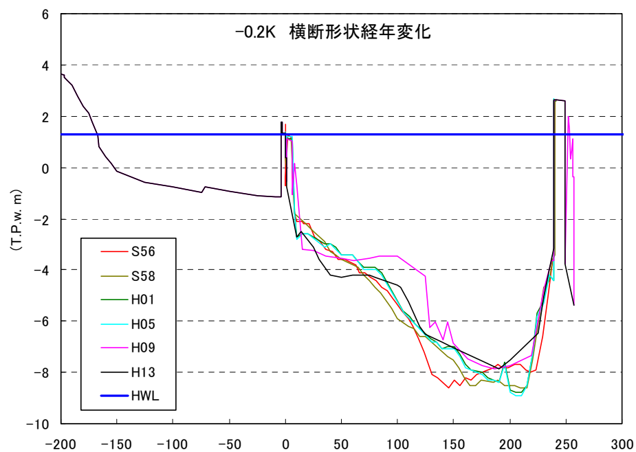
図3-2 河口部 (-0.2k) の横断図
