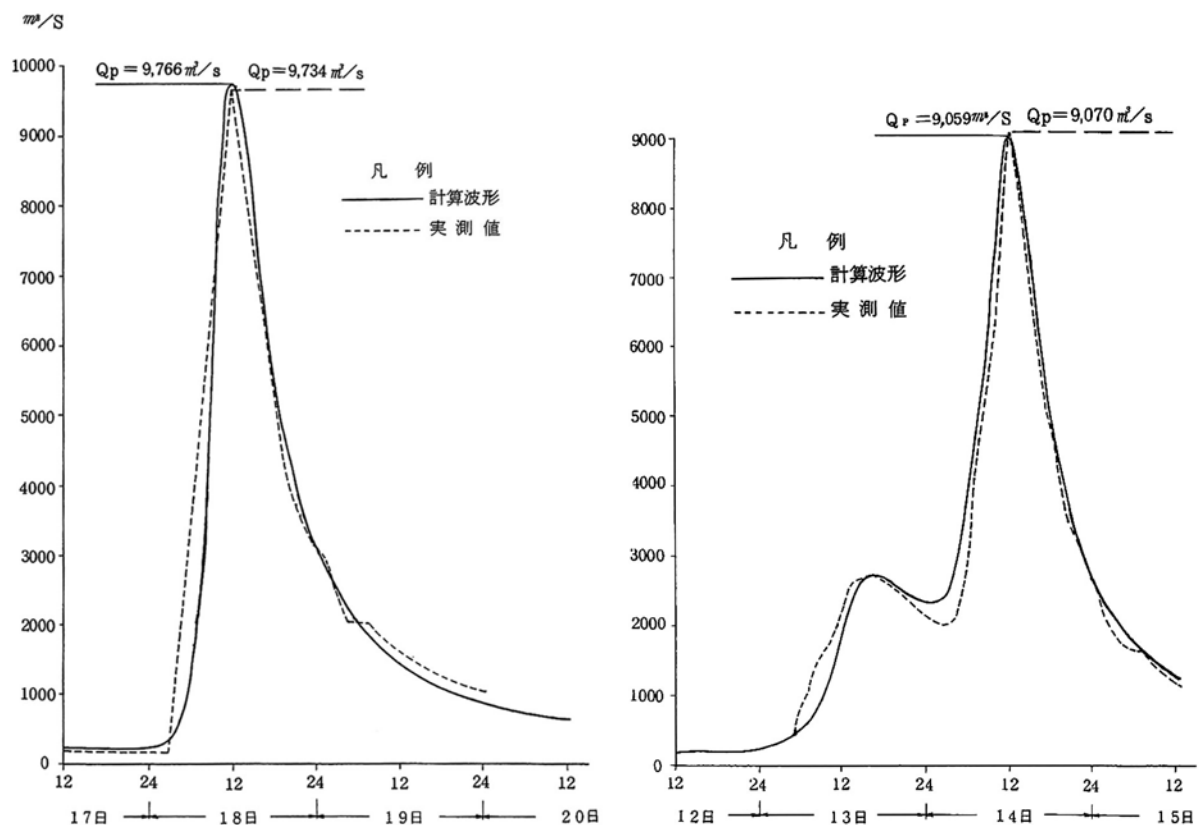
図 4-5 再現計算結果（八斗島地点）
