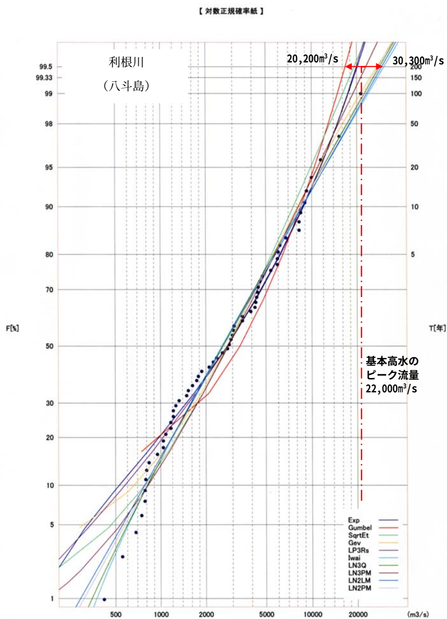
図 4-14 利根川・八斗島地点流量確率図
