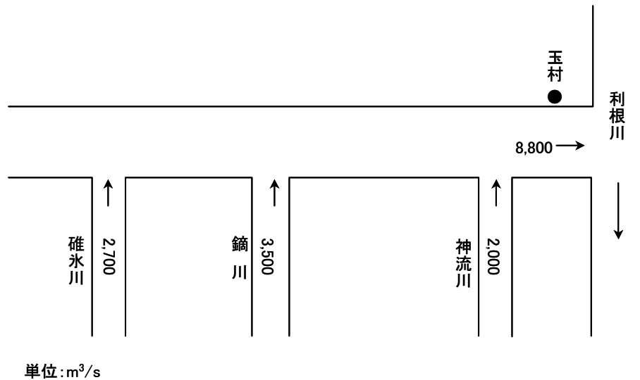
図 6-1 (2) 烏・神流川計画高水流量図
