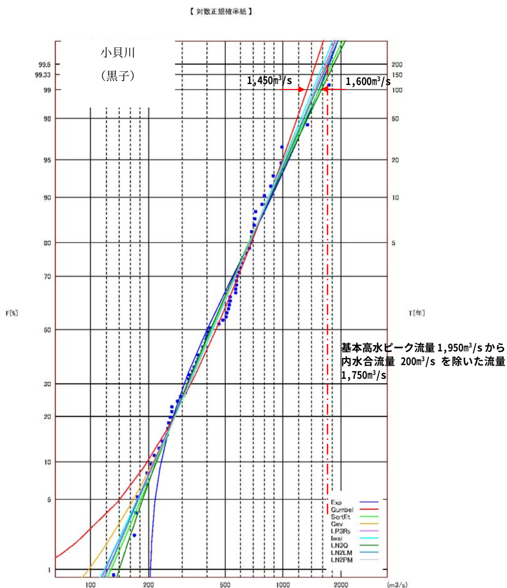
図 4-17 小貝川・黒子地点流量確率図
