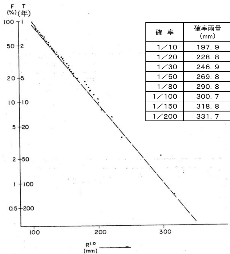
図 4-4 黒子基準地点における雨量確率図
