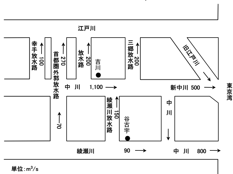
図 6-1 (7) 中川計画高水流量図
