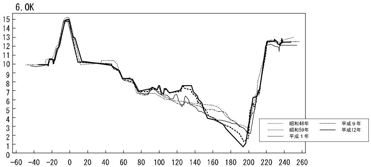
図 2-3(2) 高津川 6.0k 横断面図
