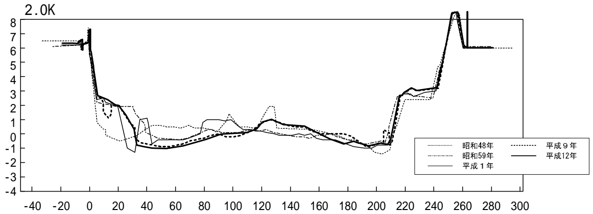
図 2-3(1) 高津川 2.0k 横断面図
