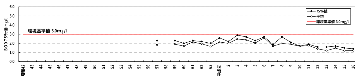
善川橋: B類型
