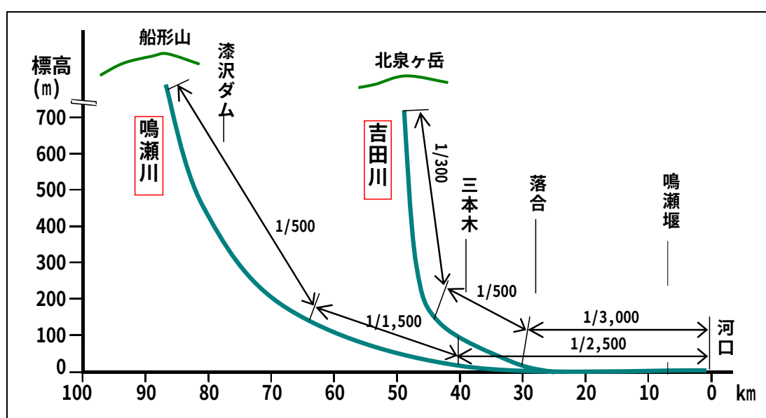
図 1-4 河川の縦断形
