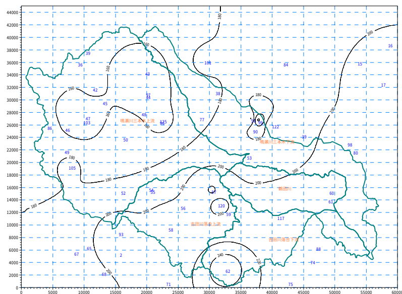
図 3-10 平成 14 年 7 月洪水等雨量線図
