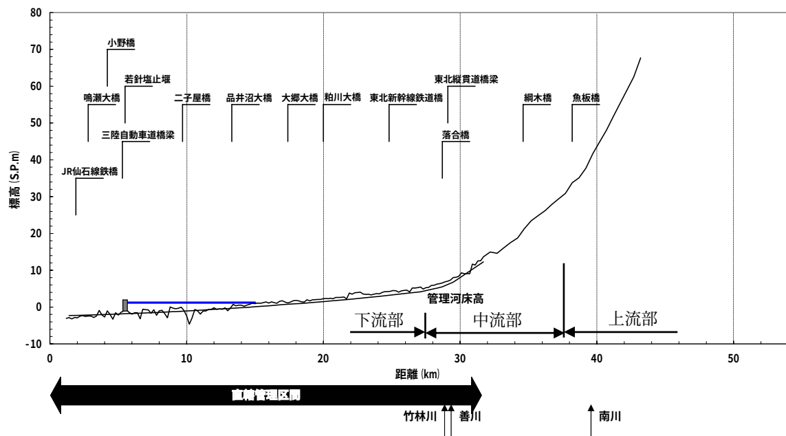
図 1-7 吉田川河道縦断図
