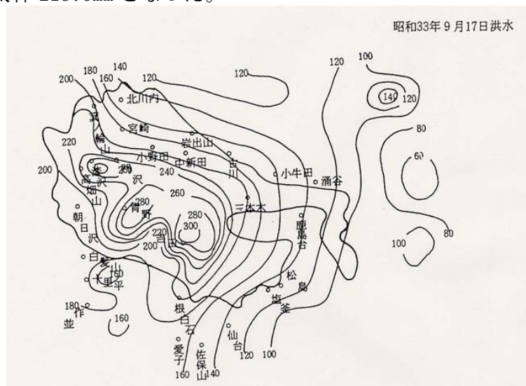
図 3-4 昭和 33 年 9 月洪水等雨量線図
