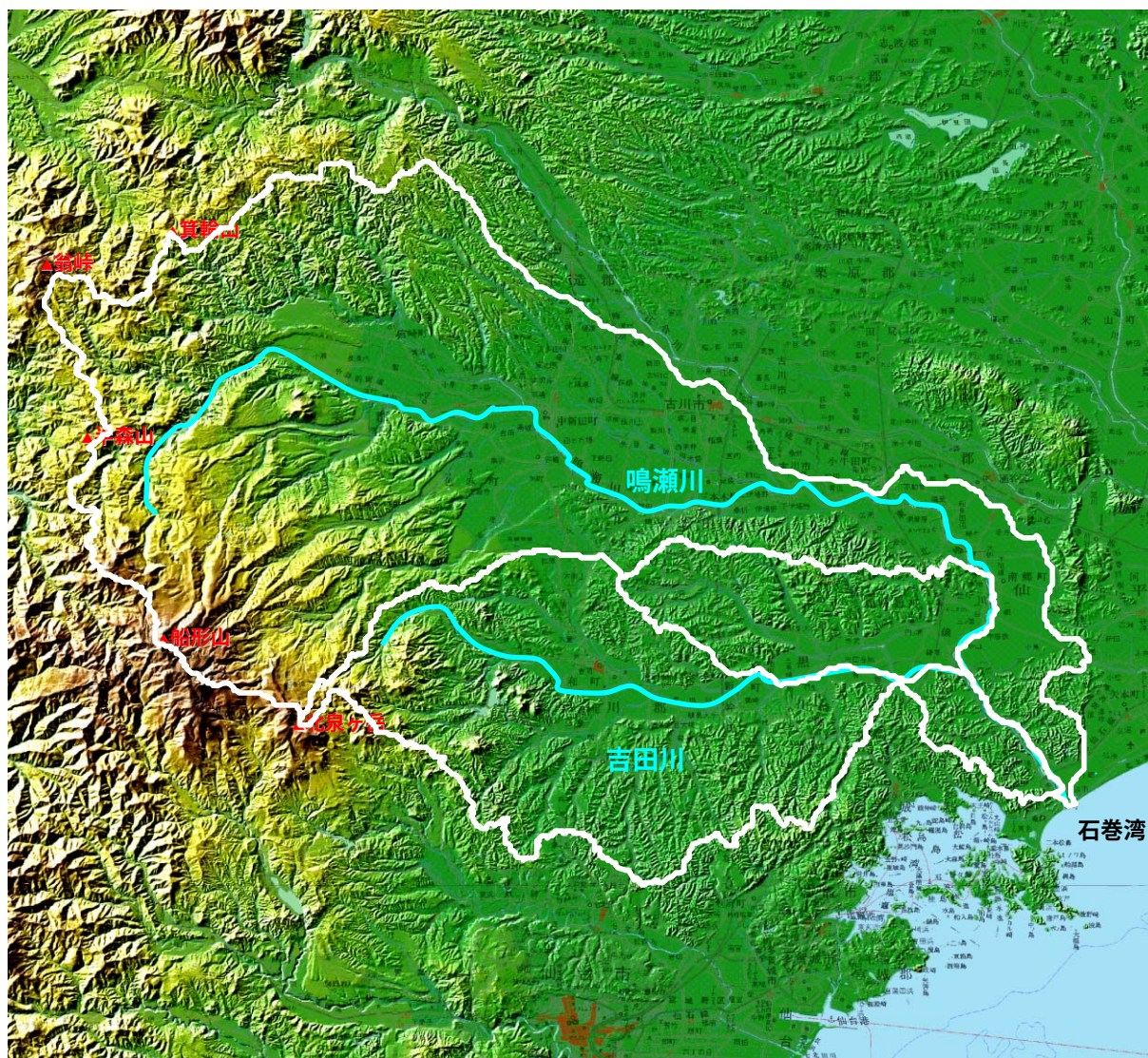
図 1-3 鳴瀬川の地形（カシミール 3D にて作成）
