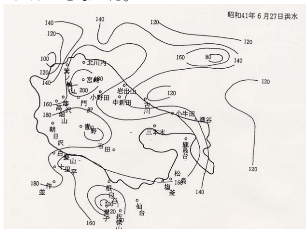
図 3-5 昭和 41 年 6 月洪水等雨量線図
