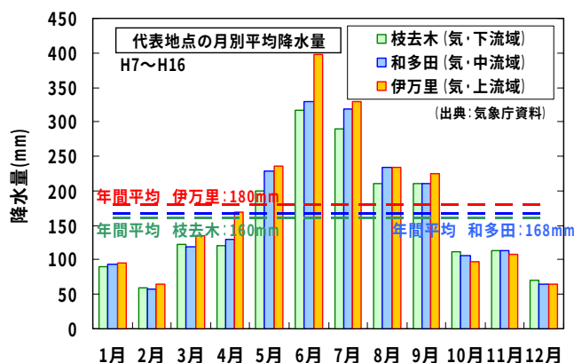
図 1- 7 代表地点の月別平均降水量
