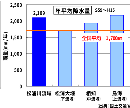
図 1- 6 年平均降水量の比較
