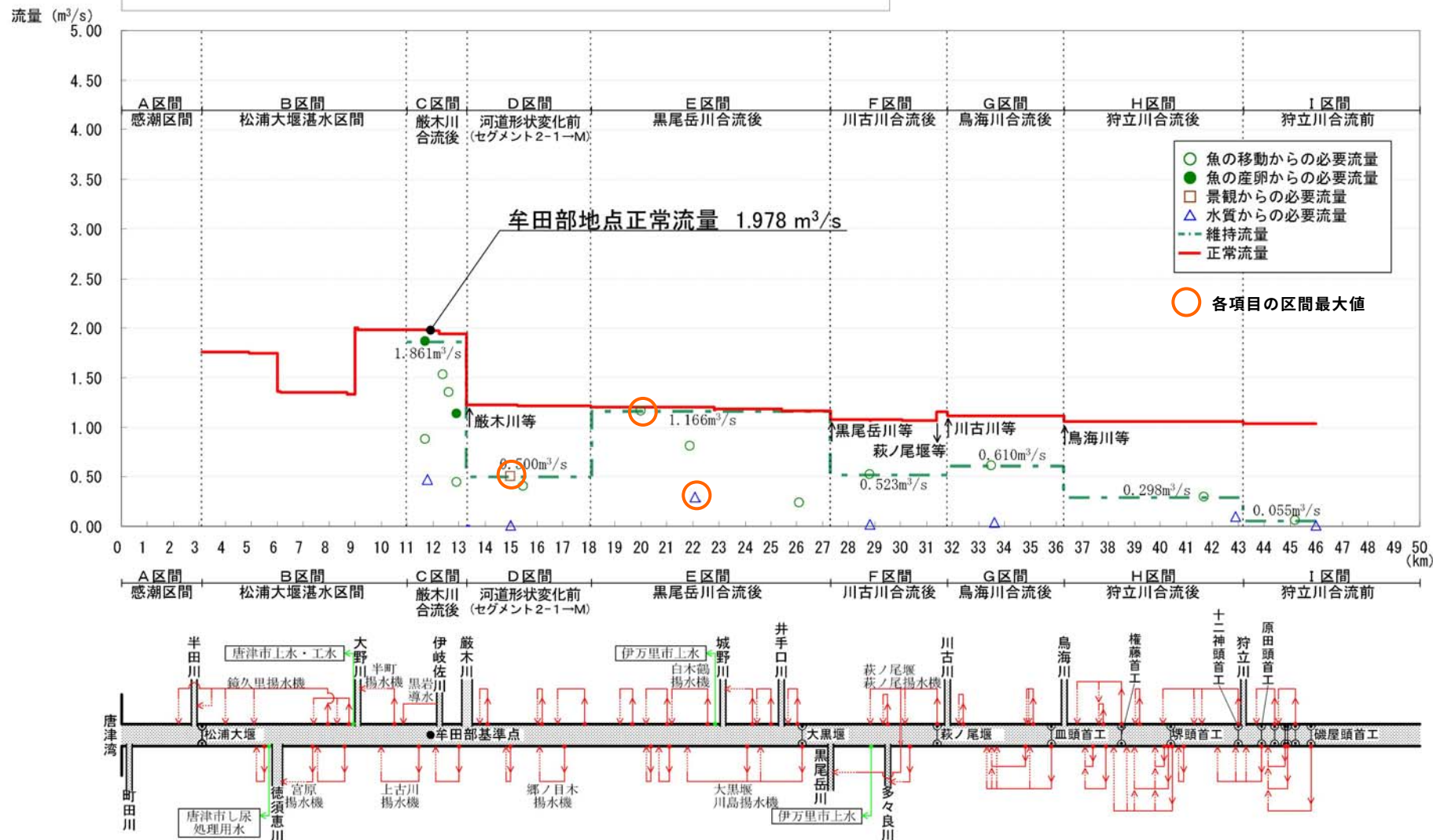
図 6-5 松浦川 正常流量縦断面図(非かんがい期 10/11~12/31)
