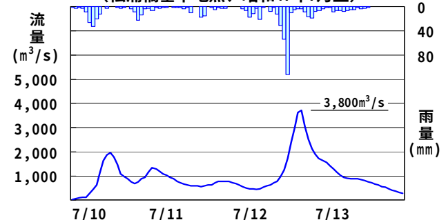
基本高水のピーク流量決定にあたり用いたハイドログラフ (松浦橋基準地点、昭和47年7月型)
