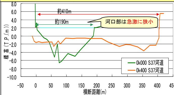
0k0地点と0k4地点の比較横断面図
