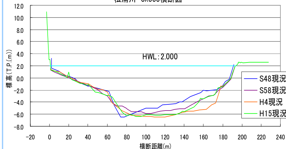
松浦川 0k000横断面図
