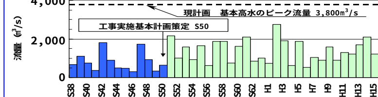
〈松浦川 松浦橋基準地点 年最大流量データ〉
