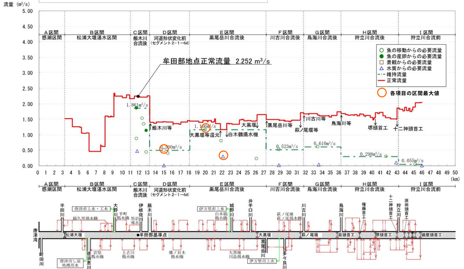
図 6 - 2 松浦川 正常流量縦断図(かんがい期 9/1~10/10)
