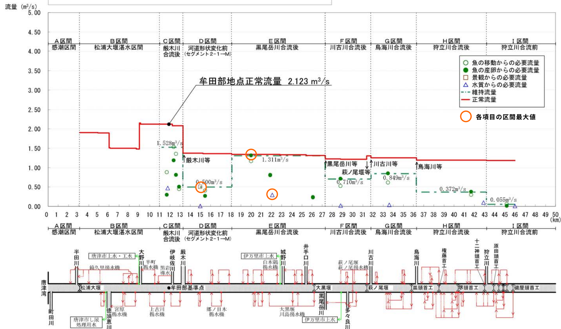
図 6-4 松浦川 正常流量縦断面図(非かんがい期 5/1~6/10)
