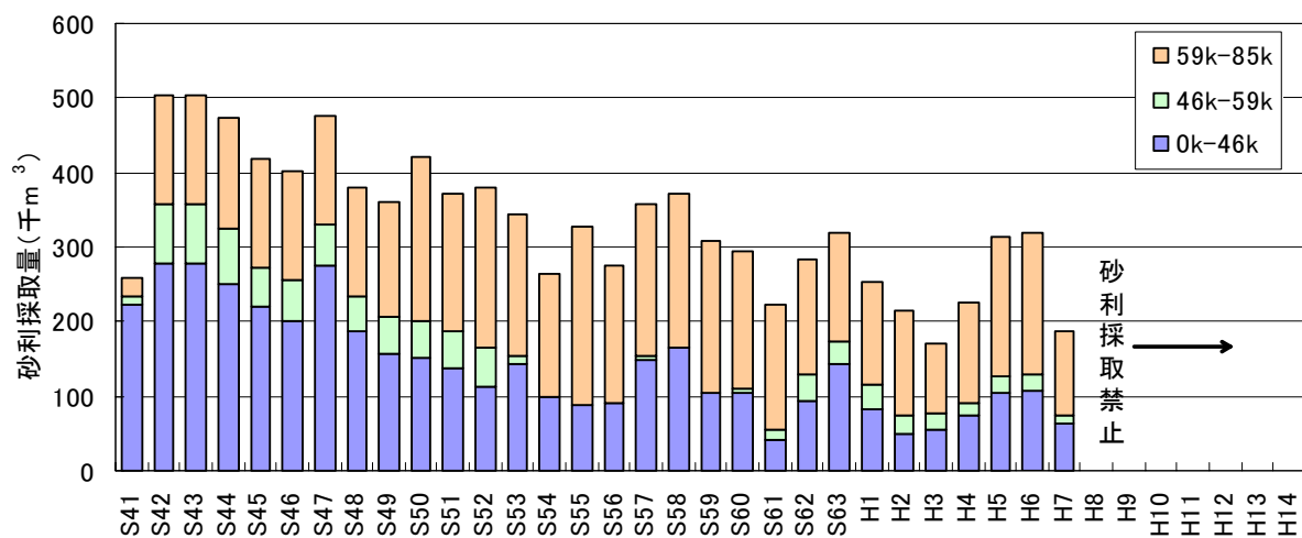
図-6 砂利採取量の経年変化図
