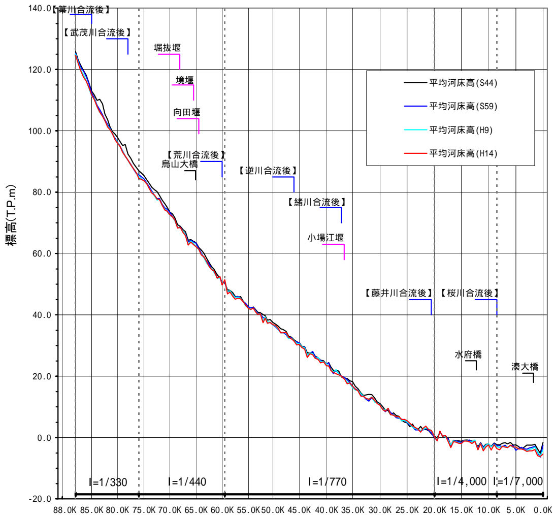
図-2 低水路平均河床高縦断図
