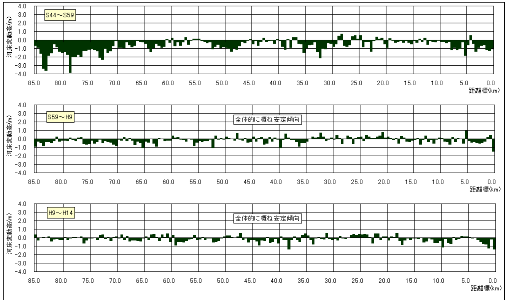
図-3 河床変動量の経年変化
