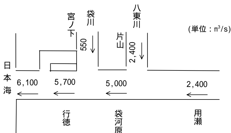
千代川計画高水流量図
