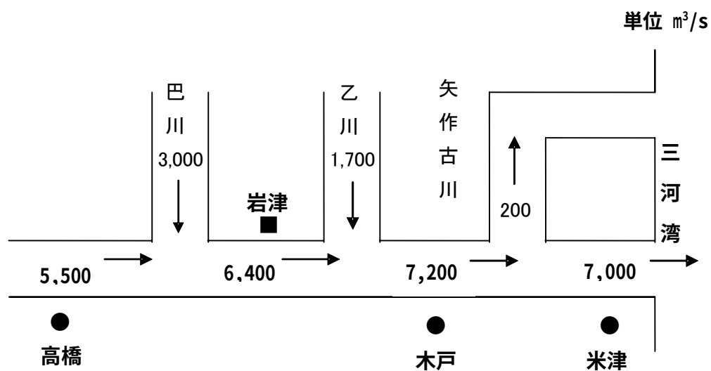
図6-1 矢作川計画高水流量図
