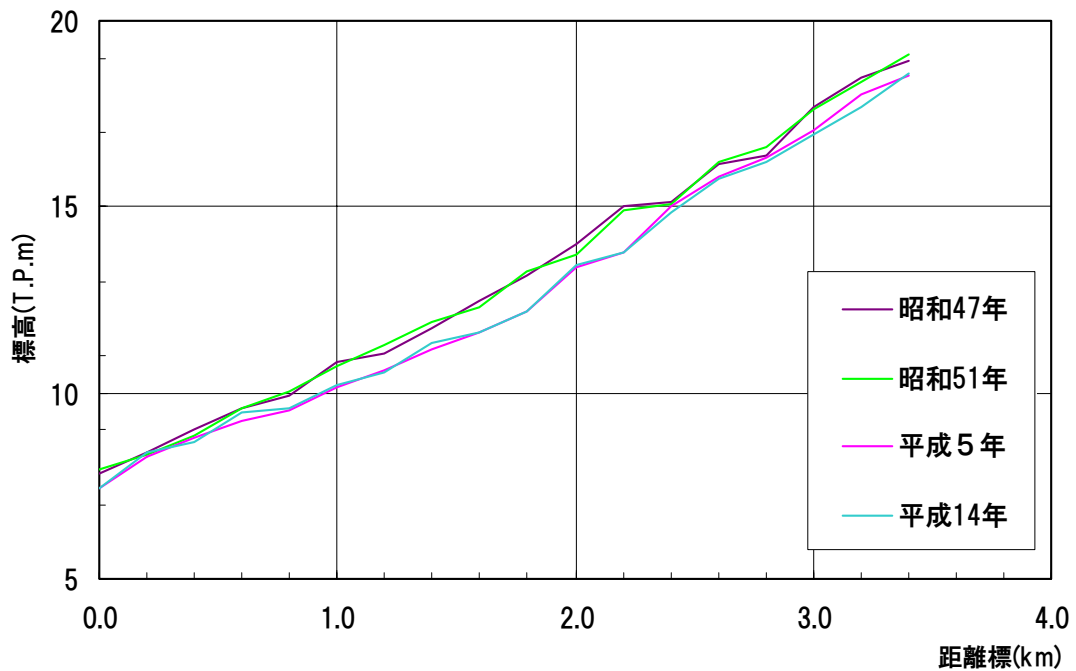
図2-5 石手川河床縦断面図
