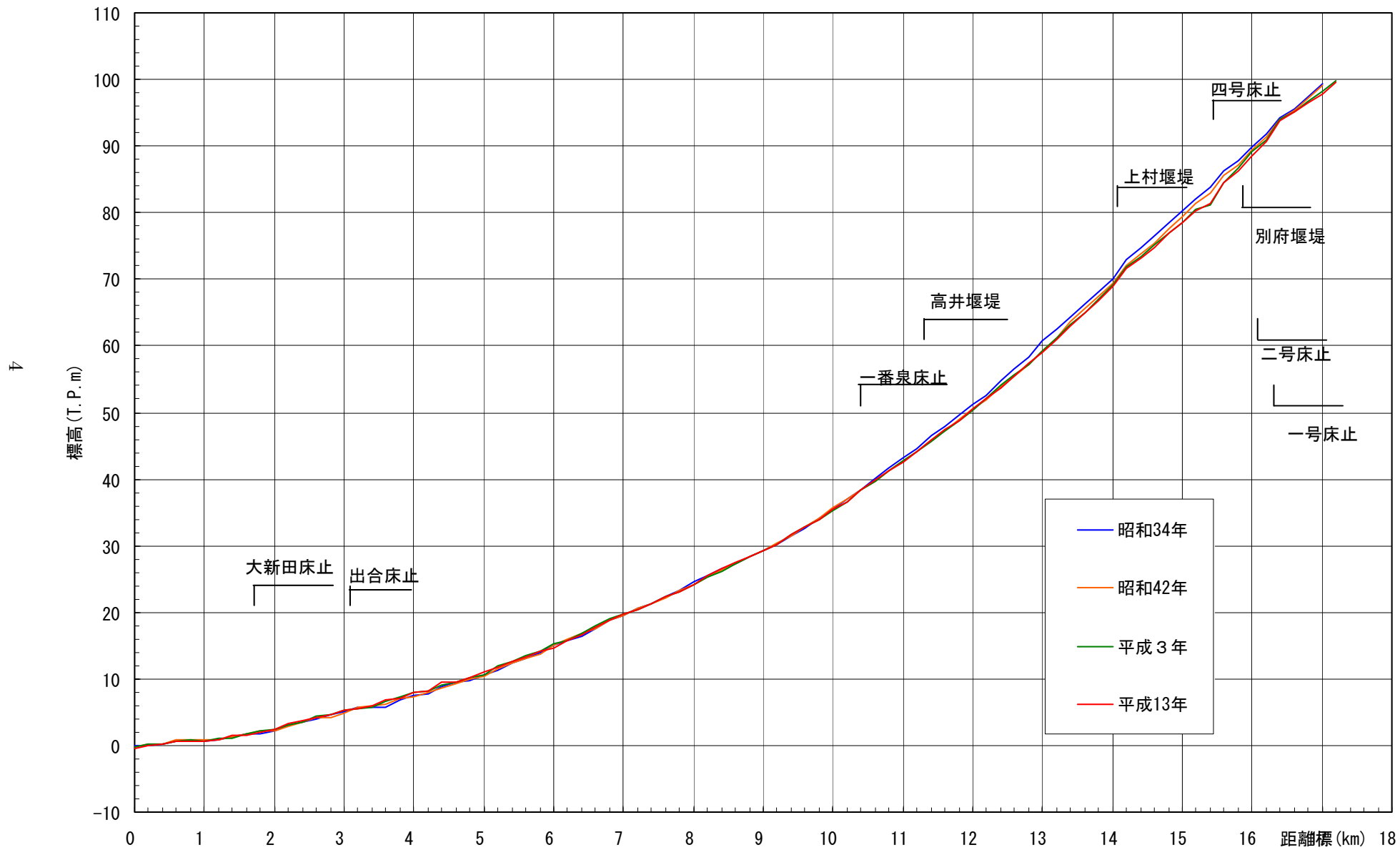
图 2 - 1 重信川河床縦断図
