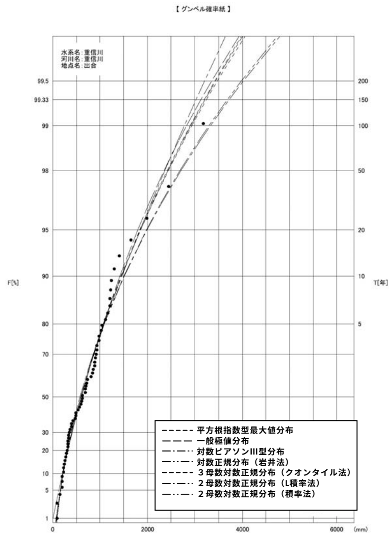
図4-11 重信川出合地点流量確率図 (昭和18年～平成16年: 62ヵ年)
