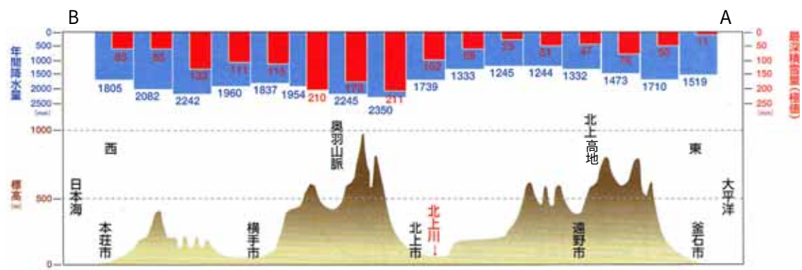
図 1-8 本荘―釜石間の横断面と年間降水量 (S28～S58)
