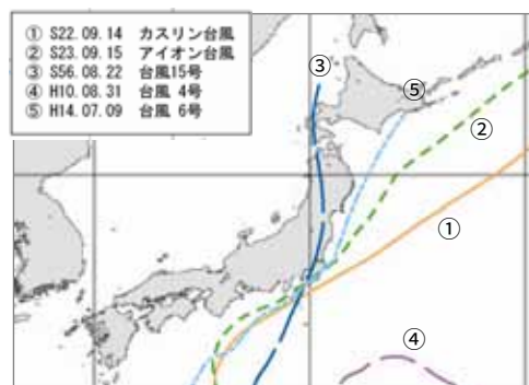
図 4-1(1) 主要洪水における台風経路図
