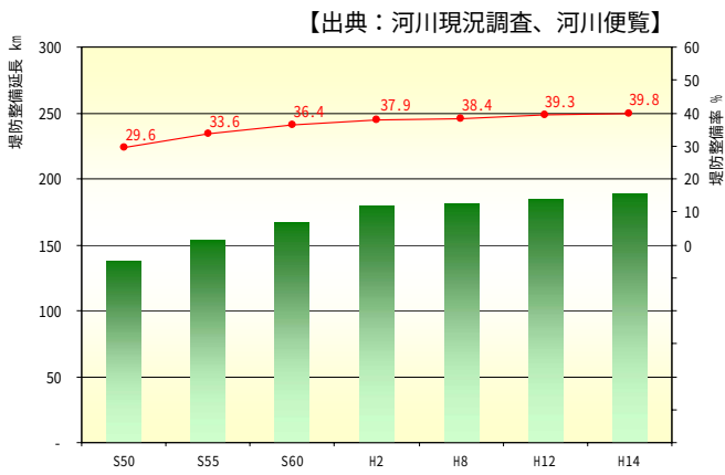
図 9-2 北上川における堤防整備状況の推移
