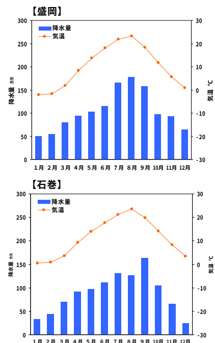
図 1-7 各地の年平均気温・降水量
