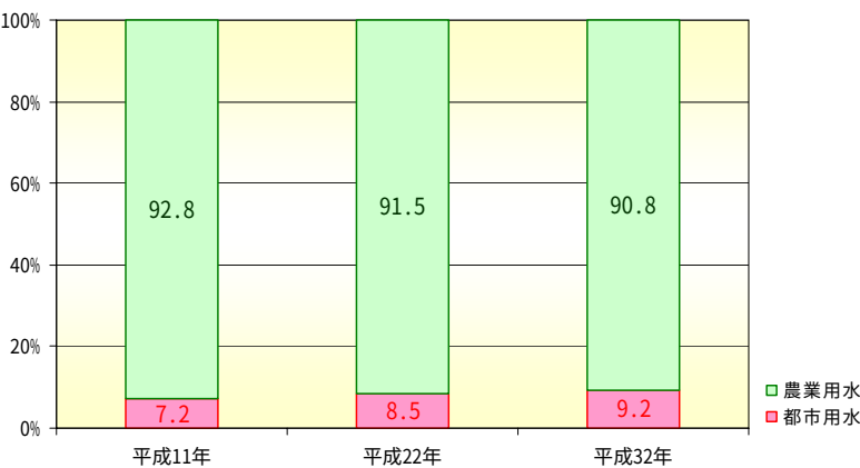
図 5-3 北上川水系（岩手県）における水需給量の推移
