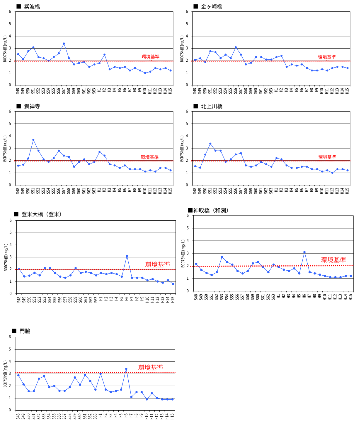
図 6-4 主要地点における水質経年変化図
