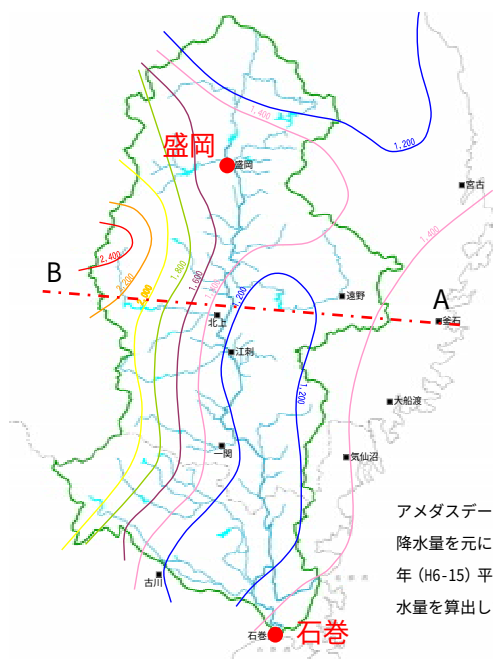
図 1-6 北上川流域 年間降水量
