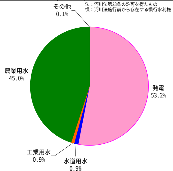
図 5-2 北上川における目的別水利流量割合
