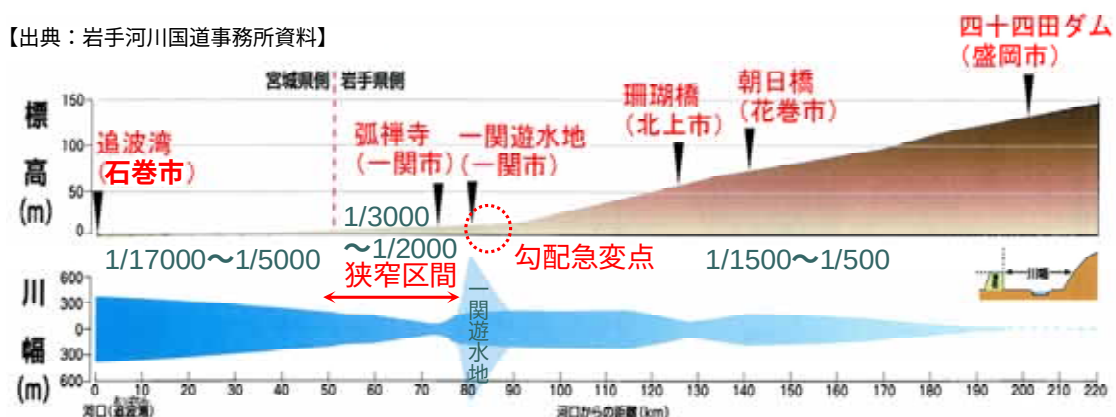
図 1-4 北上川の勾配と川幅
