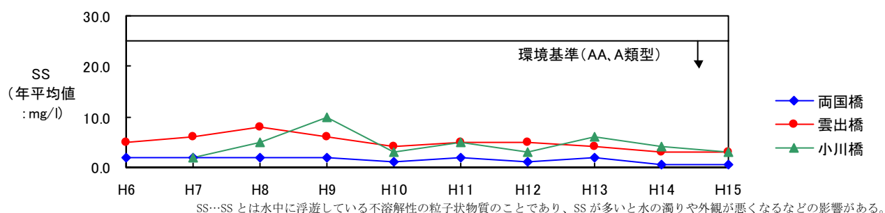
図 6-6 雲出川水質経年変化（SS）
