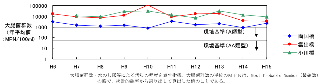
図 6-5 雲出川水質経年変化（大腸菌群数）
