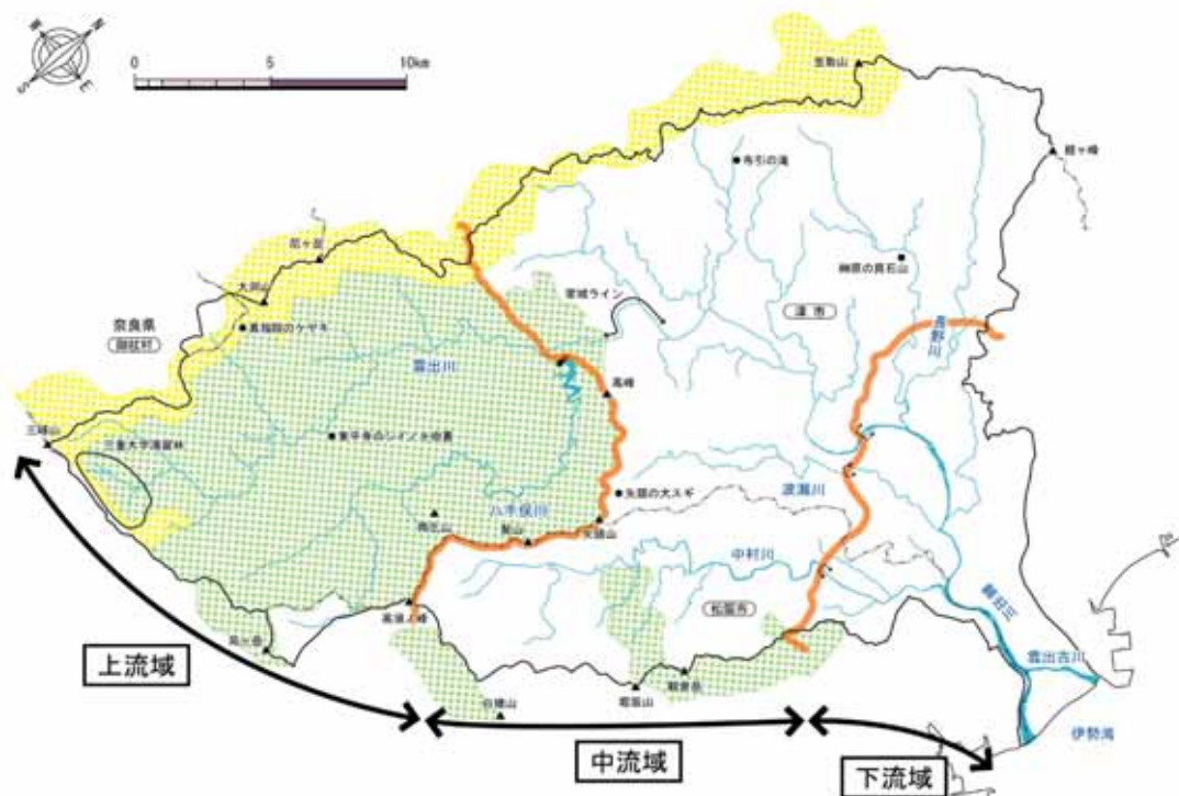
図 2-1 流域区分図
