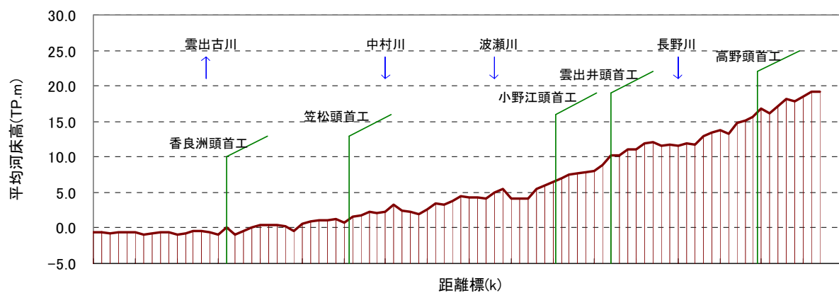
図 8-2 雲出川縦断図（大臣管理区間）
