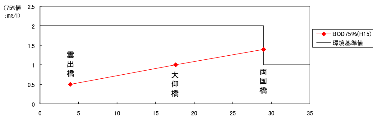
図 6-7 雲出川水質縦断変化 BOD75%値（H15 年度）
