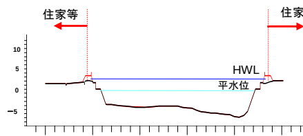
石巻市内河道断面(3.0k付近)
