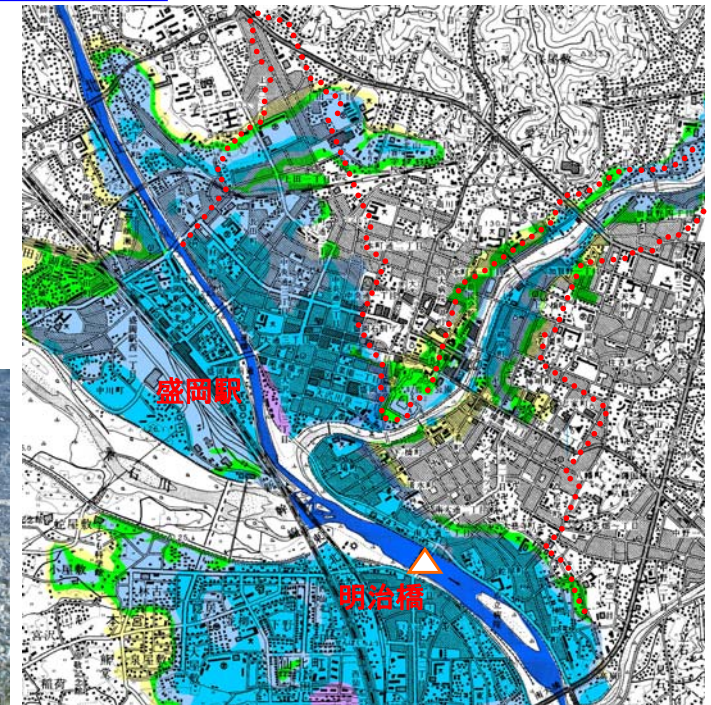
盛岡市街地における浸水想定区域図 ..... 明治43年9月洪水における浸水域
