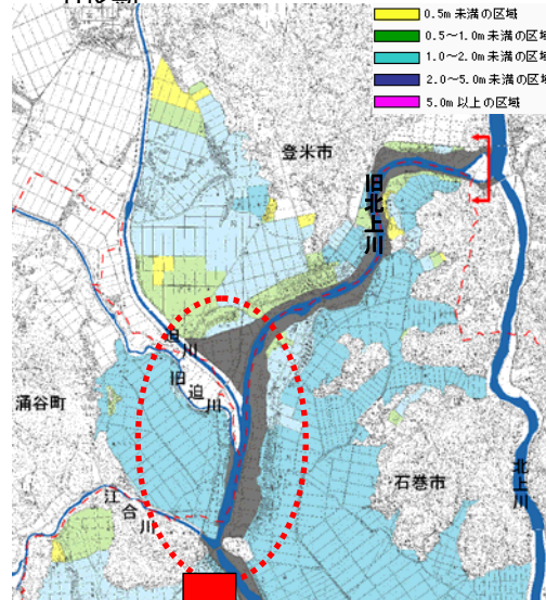
迫川付近の浸水想定区域図
