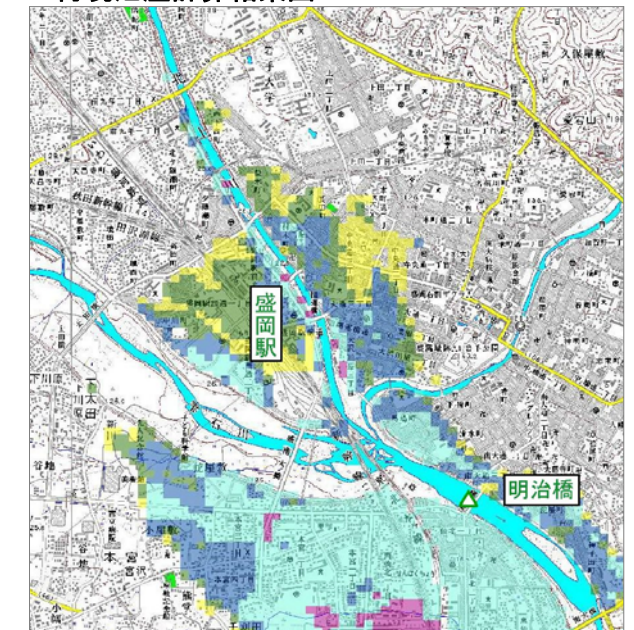
氾濫計算結果浸水区域図
