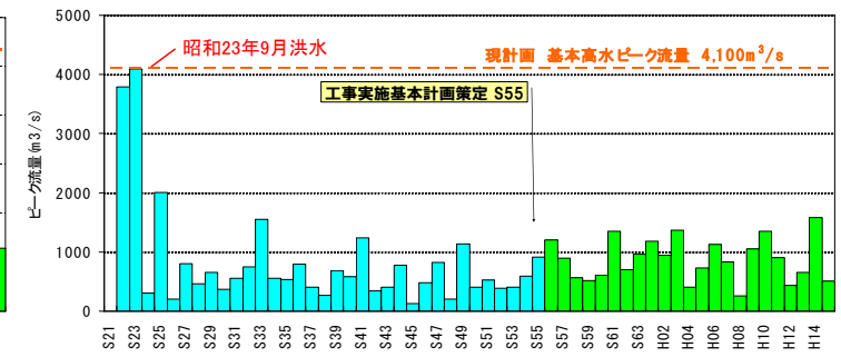
和渚地点 年最大流量データ
