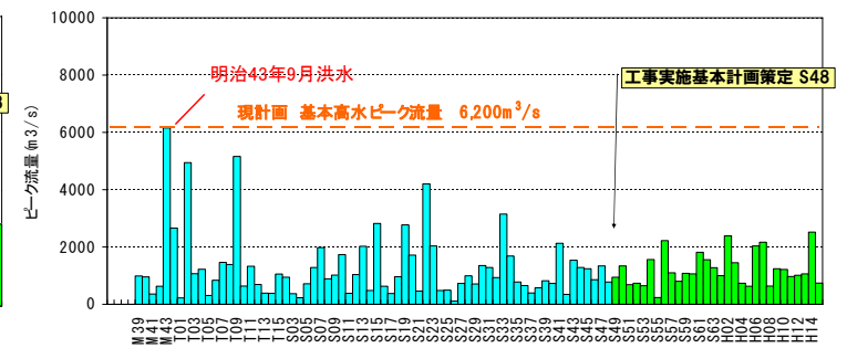
明治橋地点 年最大流量データ
