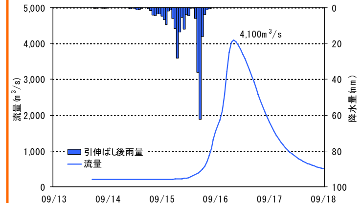
基本高水のピーク流量を決定する際に用いたハイドログラフ
