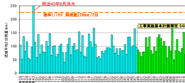
明治橋地点 年最大2日雨量データ
