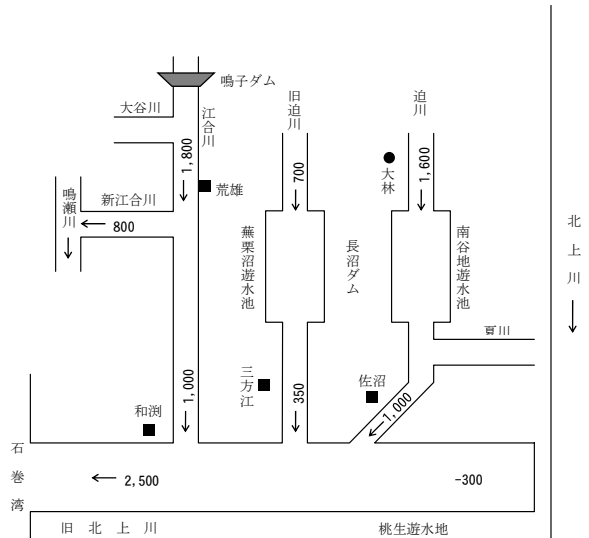
旧北上川流量配分図
