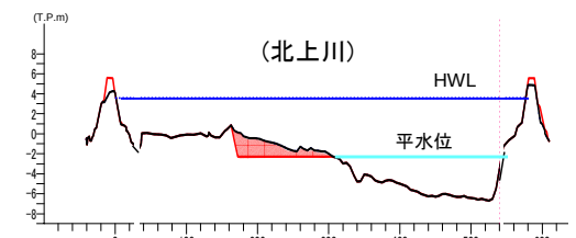
石巻市内河道断面(3.2k付近)
