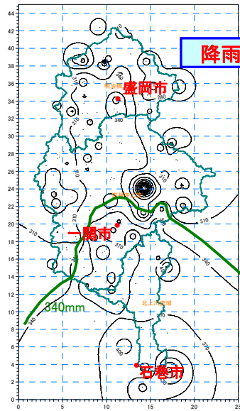
平成14年7月洪水 等雨量線図
