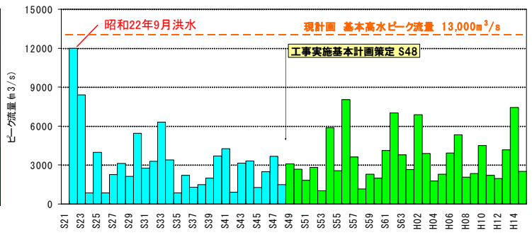
狐禅寺地点 年最大流量データ
