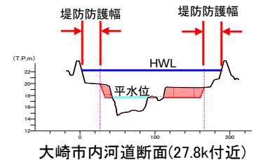
大崎市内河道断面(27.8k付近)
