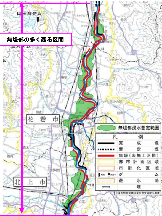
中流部の無堤状況
