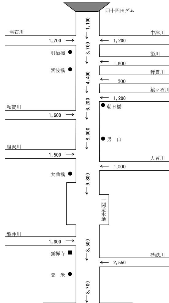
北上川流量配分図
