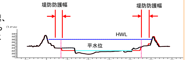
奥州市内河道断面(44.4k付近)
