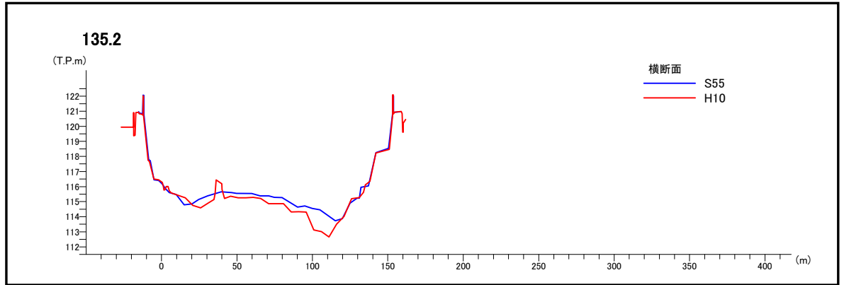
図 2-4(1) 明治橋付近の横断面図
