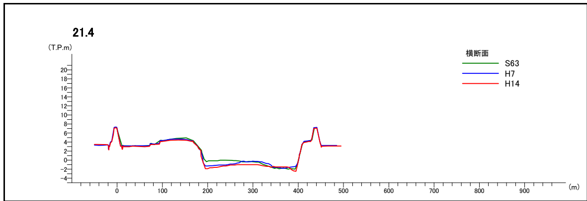
図 2-5 和湊付近の横断面図
