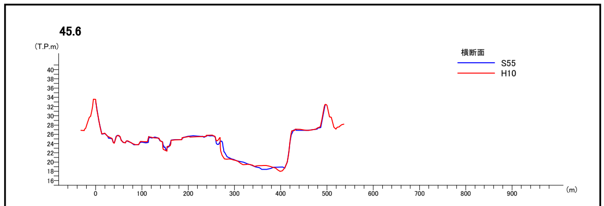
図 2-4(2) 大曲橋付近の横断面図
