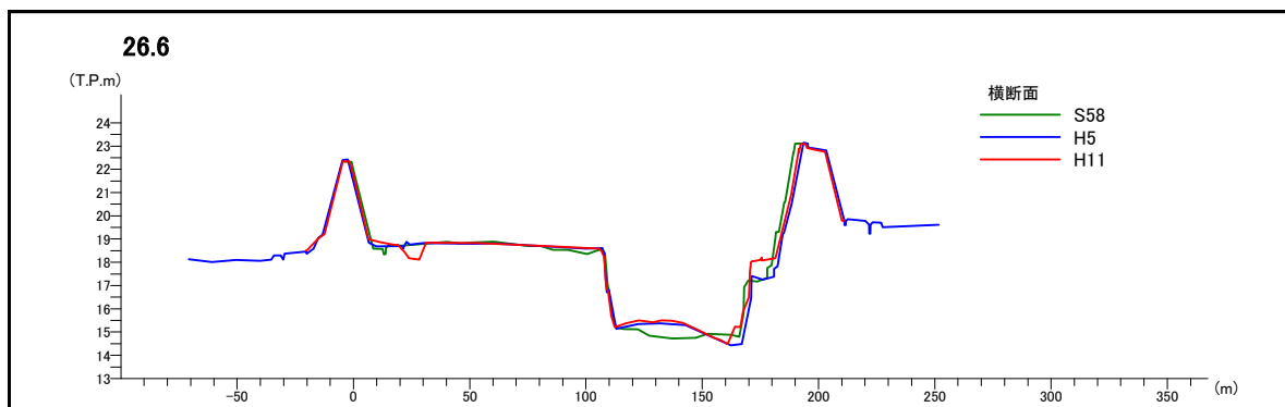
図 2-6(1) 荒雄付近の横断面図
