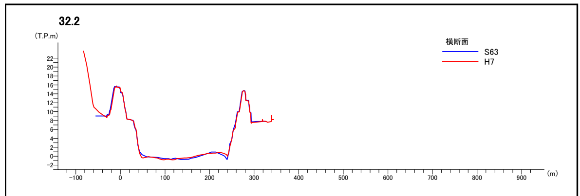
図 2-4(3) 登米付近の横断面図
