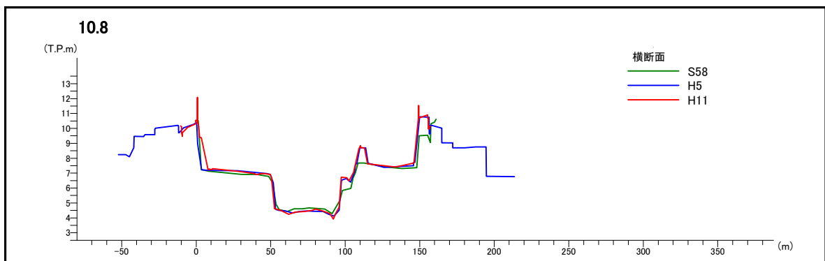
図 2-6(2) 涌谷付近の横断面図
