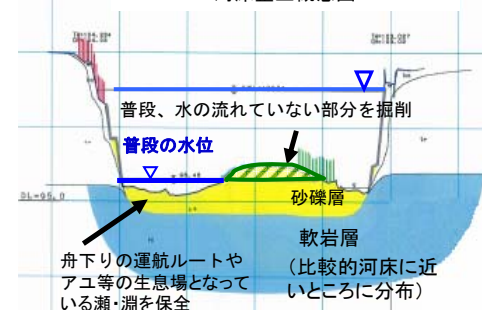
河床掘削概念図
