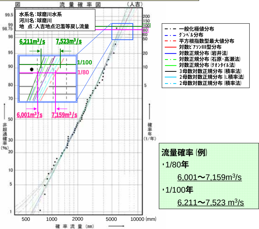
球磨川水系流量確率計算結果(基準地点: 人吉、対象年: 昭和28年～平成17年)
