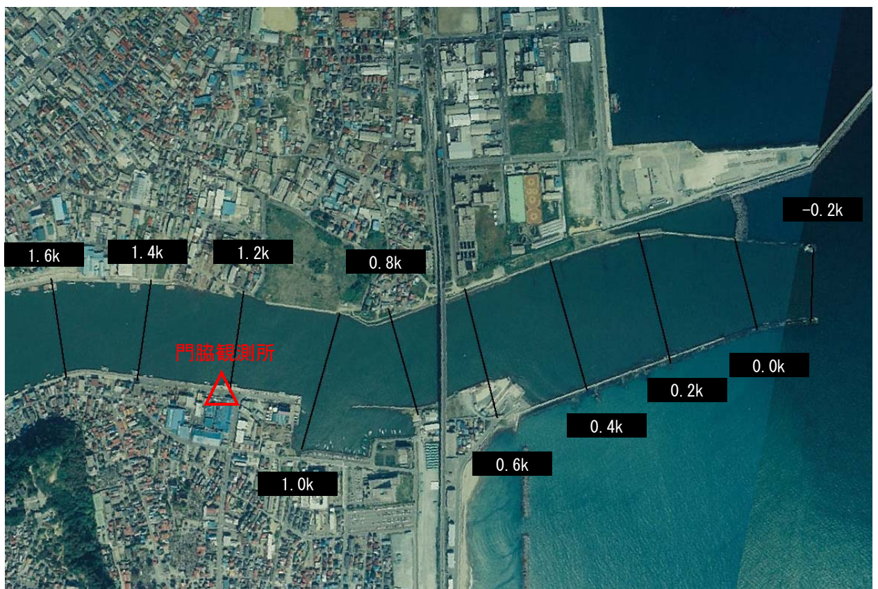
図 3-3 平面図 (旧北上川)
