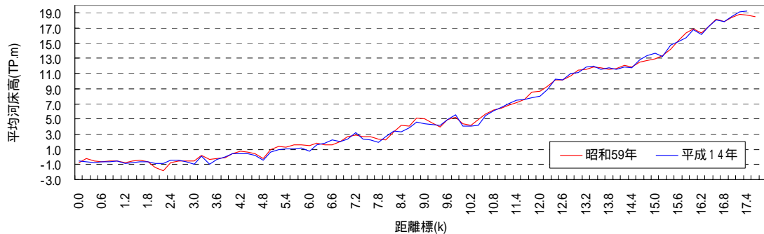
図 2.5 縦断変遷図（雲出川本川）
