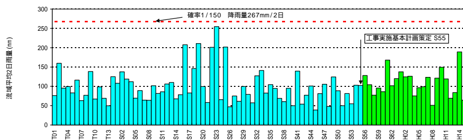
図 4-5 (4) 年最大2日雨量 (旧北上川和湊地点上流)
