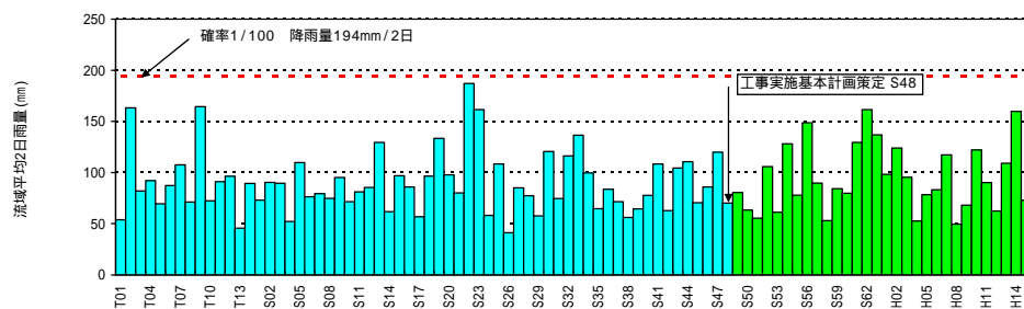
図 4-5 (2) 年最大2日雨量 (北上川狐禅寺地点上流)
