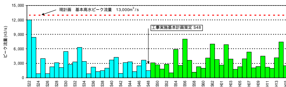
図 4-5 (1) 年最大流量 (ダム・氾濫戻し流量、北上川狐禅寺地点)
