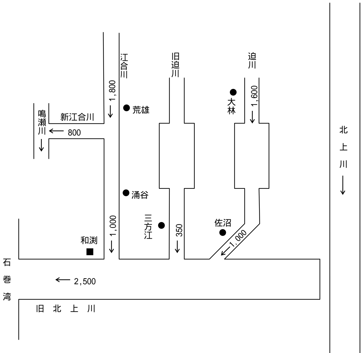
図 6-2 計画流量配分図 (旧北上川)
