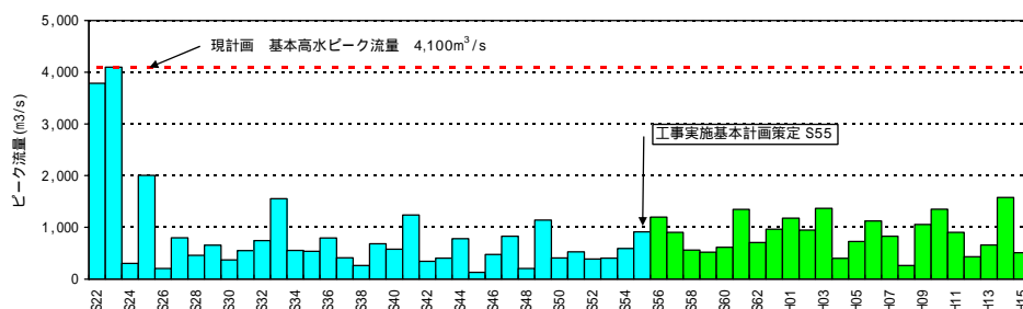
図 4-5 (3) 年最大流量 (ダム・氾濫戻し流量、旧北上川和湊地点)
