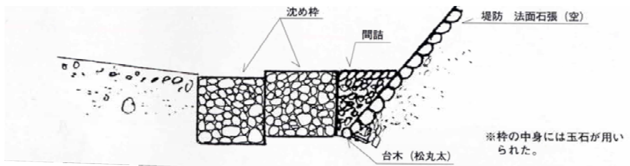
図 4-4 沈め枠
