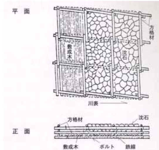
図 4-6 木工沈床
