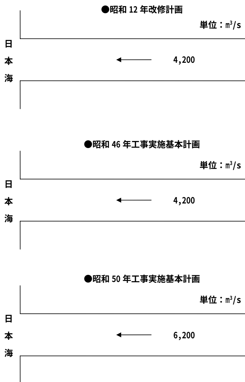
図 4-3 計画高水流量の変遷（河道配分図）
