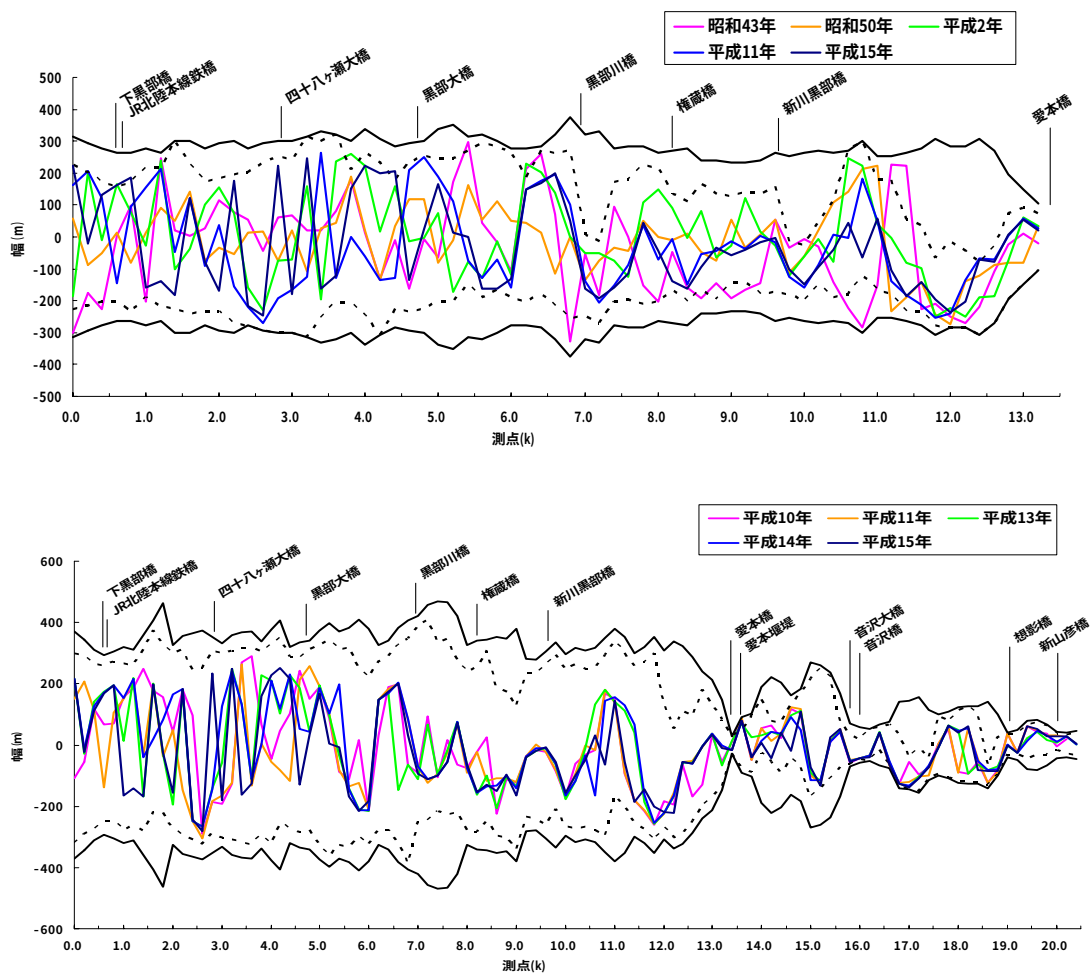
図 4-14 滞筋の変遷
