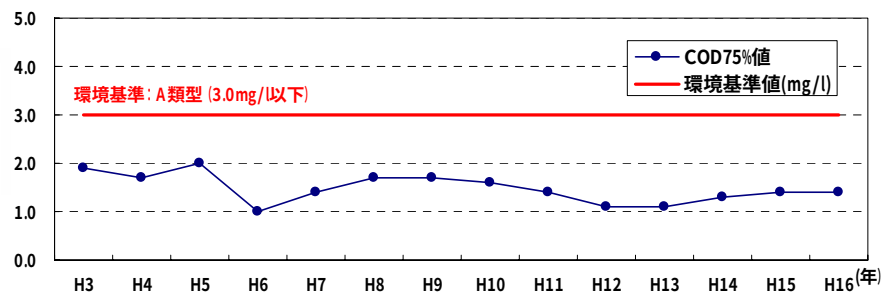
水質経年変化図（黒部ダム貯水池堰堤付近）COD
