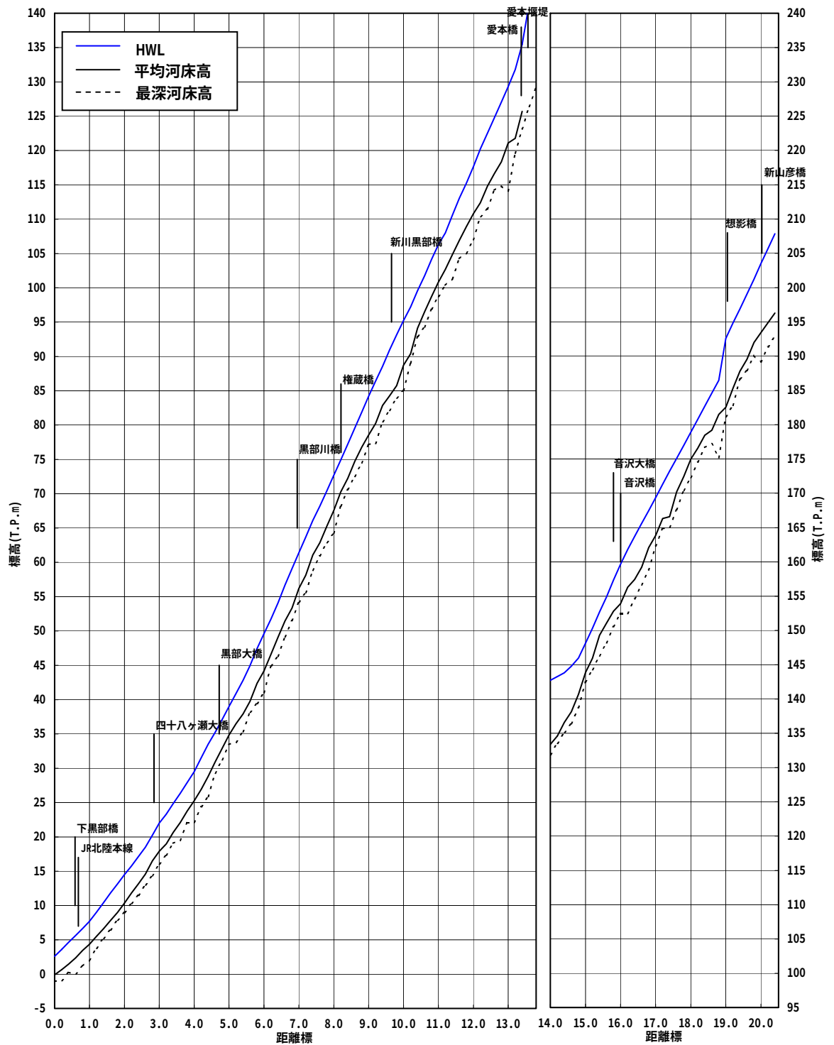
図 8-2 黒部川現況(H15)河道縦断面図（直轄管理区間、ダム管理区間除く）
