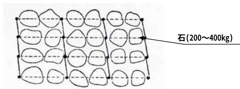
図 4-5 連石床
