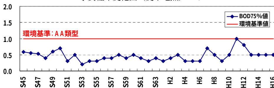
水質経年変化図（愛本地点）BOD
