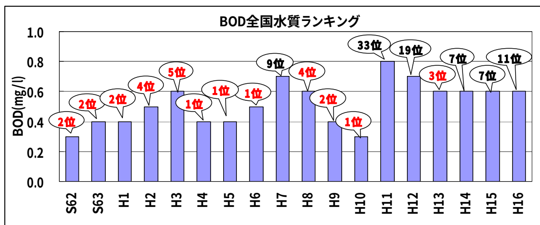
図 6-3 黒部川の水質（BOD）と全国水質ランキング
