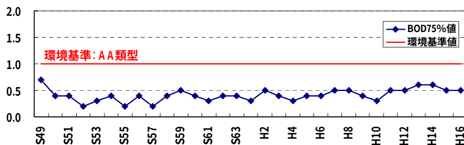
水質経年変化図（宇奈月地点）BOD
