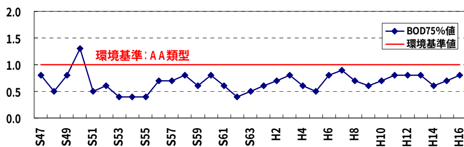
水質経年変化図（下黒部地点）BOD
