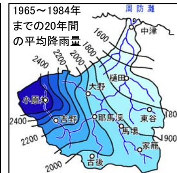
年平均降雨量分布
