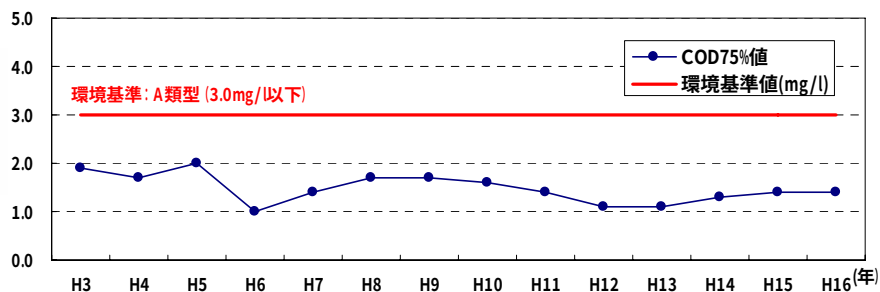
水質経年变化図（黒部ダム貯水池堰堤付近）COD
