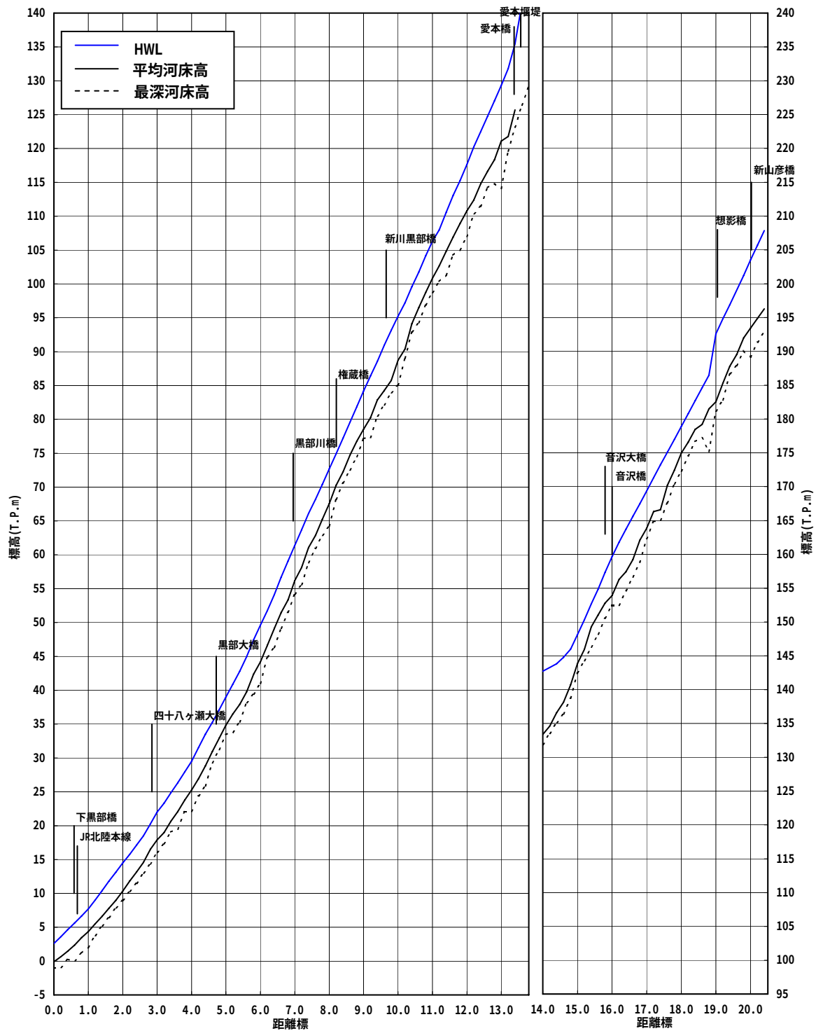
図 8-2 黒部川現況(H15)河道縦断面図（直轄管理区間、ダム管理区間除く）
