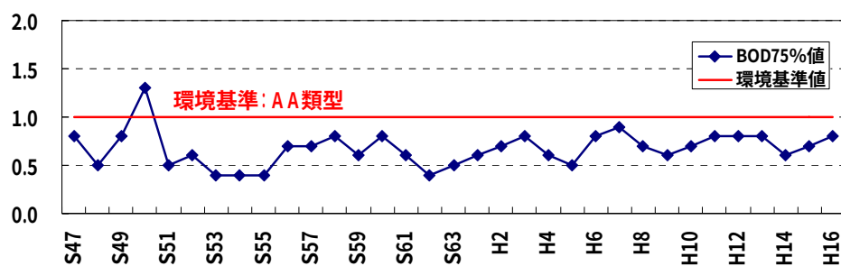
水質経年变化図（下黒部地点）BOD
