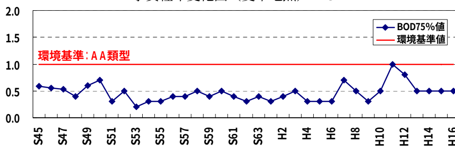
水質経年变化図（愛本地点）BOD
