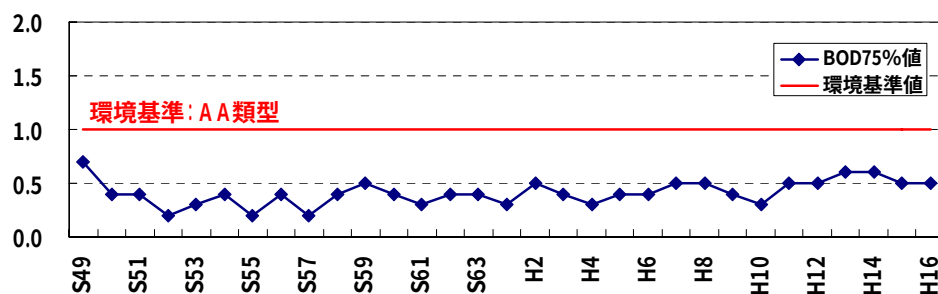
水質経年变化図（宇奈月地点）BOD
