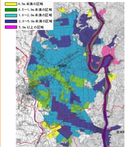
登米市 (旧中田町) 付近の浸水想定区域図
