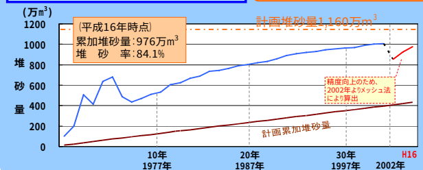
四十四田ダムの堆砂状況
