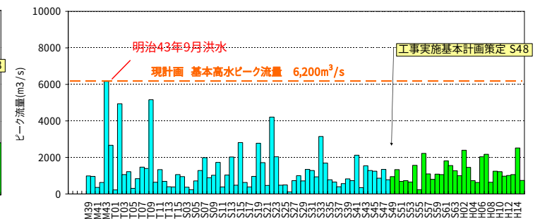
明治橋地点 年最大流量データ
