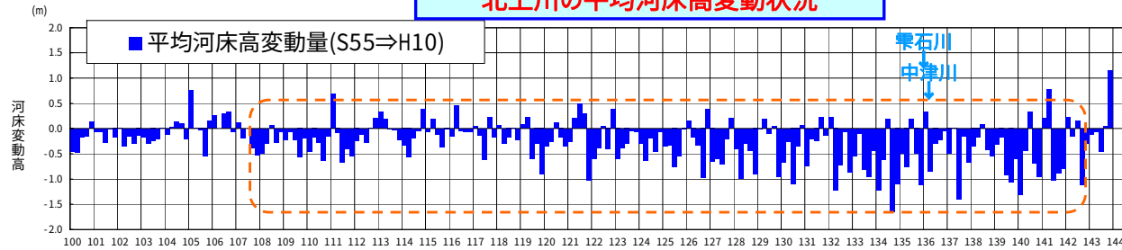
北上川の平均河床高変動状況
