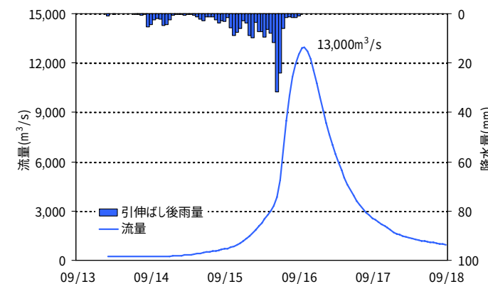
基本高水のピーク流量を決定する際に用いたハイドログラフ
